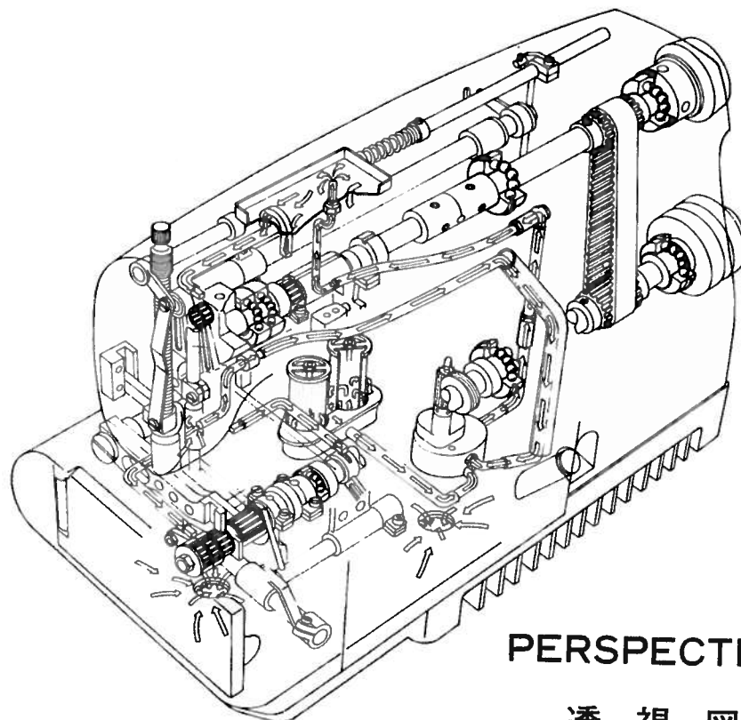
透視図
