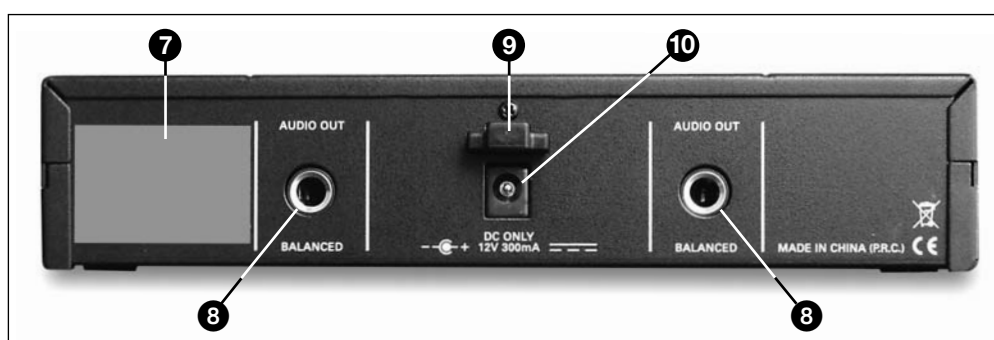
Fig. 2: Commandes de la face arrière du récepteur SR 40 DUAL
