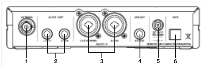
Fig. 3: Ingressi e uscite sul retro del trasmettitore
