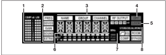
Fig. 2 : Ecran sur le panneau avant de l'émetteur
