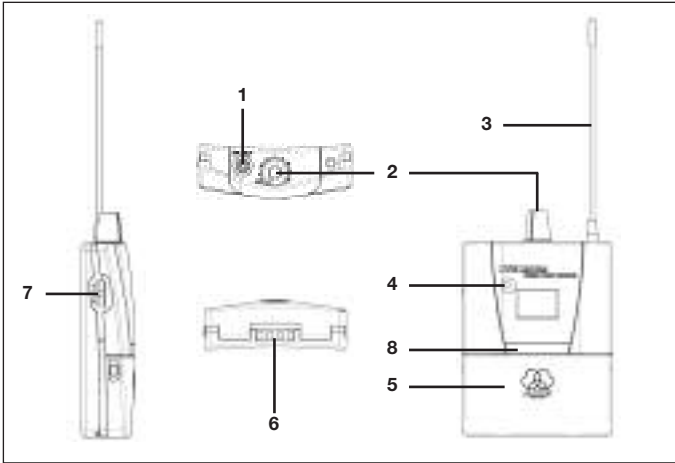
Fig. 4: Ricevitore da tasca SPR 4
