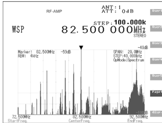
WSP Display
