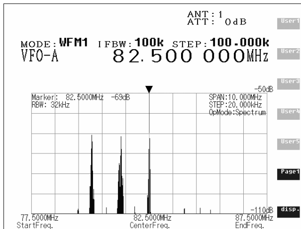
VFO mode
