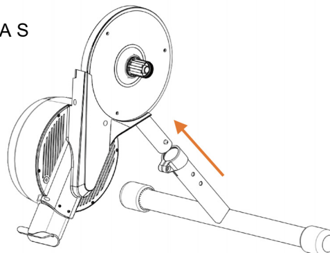
Supporto anteriore
