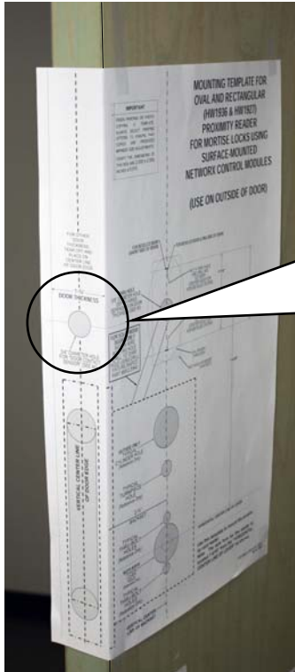
FIG. 5: DOOR CONTACT SENSOR HOLE ON DOOR EDGE
