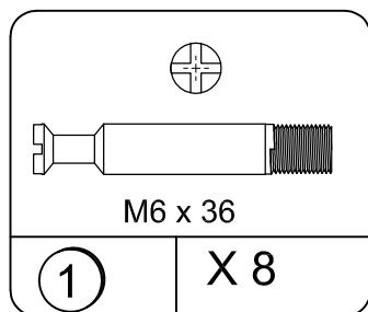
CAM BOLT Leva de Perno TWF4430
