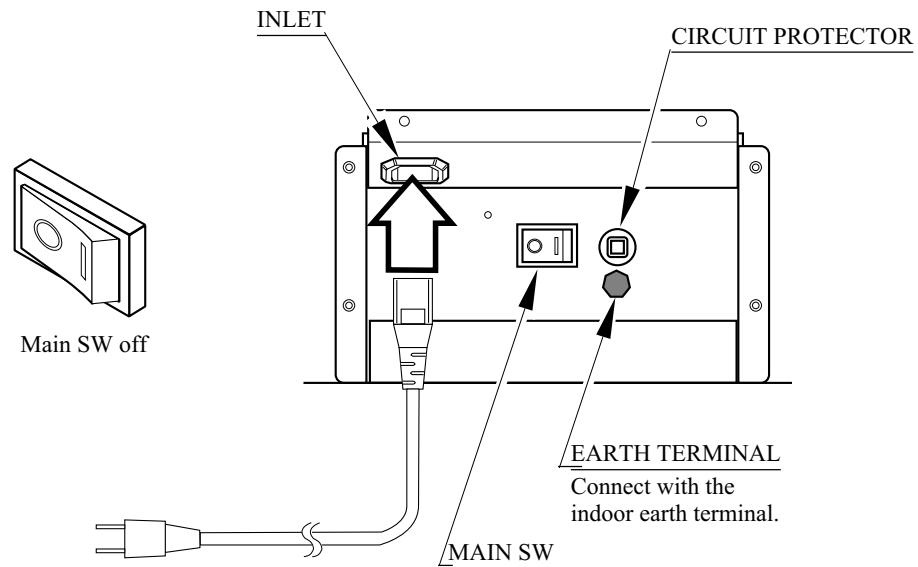
FIG. 5. 6 a AC unit
