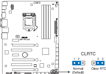
Jumper d'effacement de la mémoire CMOS de la Z87-PLUS
