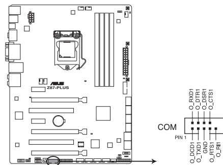
Connecteur pour port COM de la Z87-PLUS
