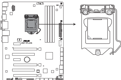
Interface de connexion LGA1150 de la Z87-PLUS
