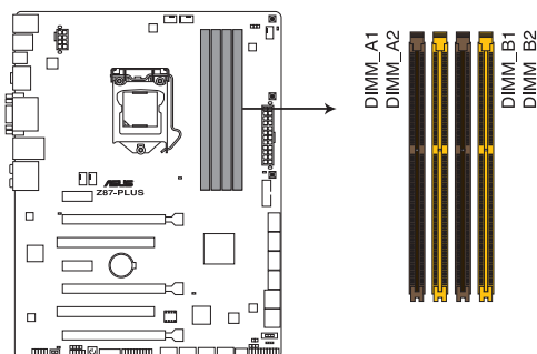
Interfaces de connexion pour modules mémoire DDR3 de la Z87-PLUS
