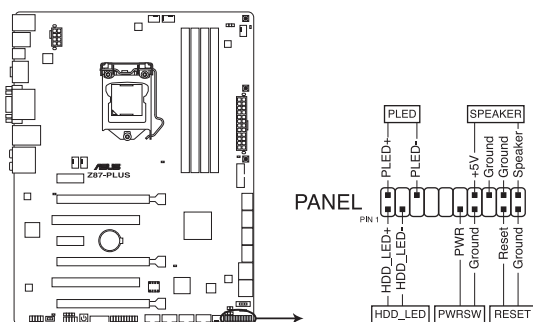
Connecteur panneau système de la Z87-PLUS
