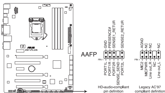
Connecteur audio pour panneau avant de la Z87-PLUS
