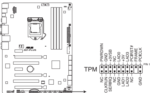
Connecteur TPM de la Z87-PLUS
