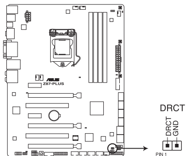
Connecteur DirectKey de la Z87-PLUS
