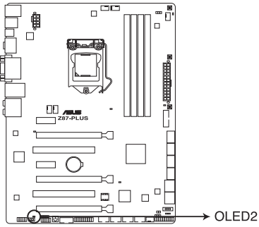
LED EPU de la Z87-PLUS
