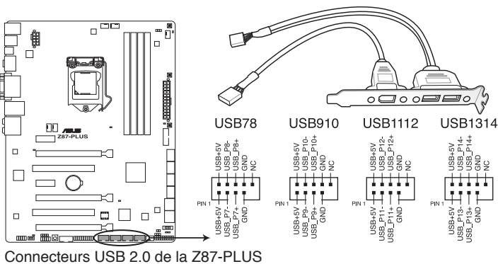
Connecteurs USB 2.0 de la Z87-PLUS
