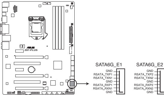
Connecteurs SATA 6Gb/s Marvell de la Z87-PLUS
