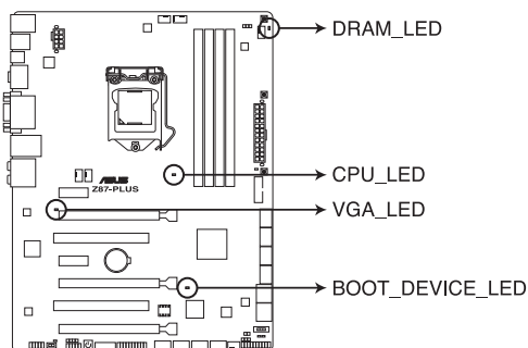
LED du POST de la Z87-PLUS
