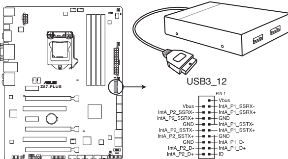
Connecteur USB 3.0 de la Z87-PLUS
