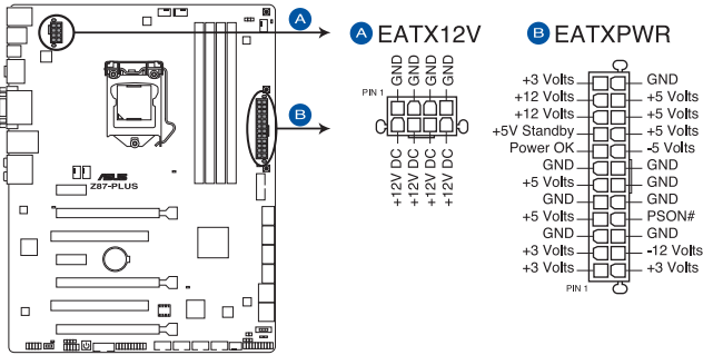
Connecteurs d'alimentation de la Z87-PLUS
