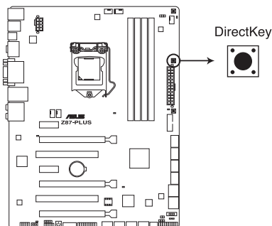
Bouton DirectKey de la Z87-PLUS
