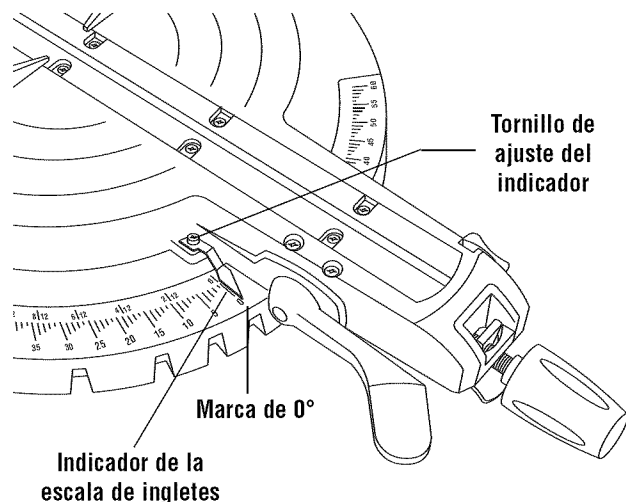
Figura 11. Ajuste de la escala de ingletes
