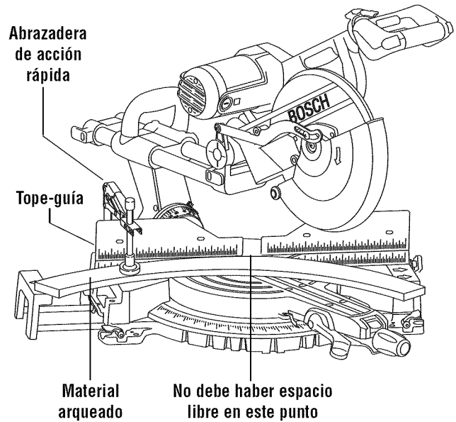
Figura 37. Material arqueado
