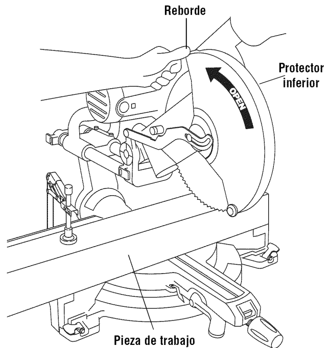
Figura 18. Subida del protector inferior
