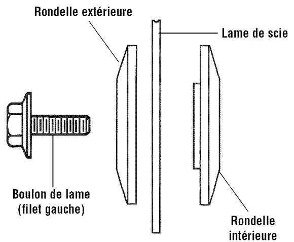
Figure 2. Ferrures de lame
