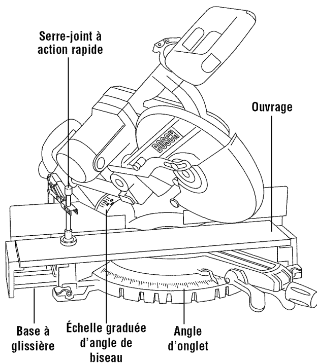
Figure 32. Coupe composée
