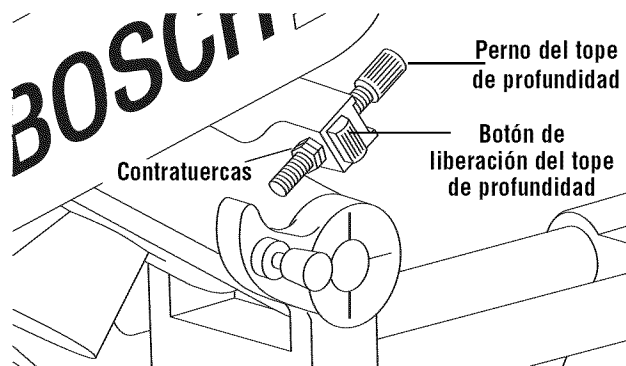
Figura 13. Ajuste de la profundidad
