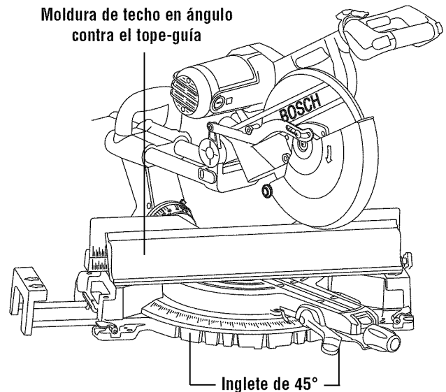
Figura 36. Moldura de techo en ángulo respecto a la mesa y al tope-guía
