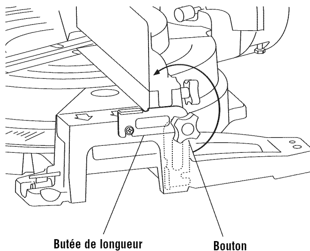
Figure 34. Butée de longueur
