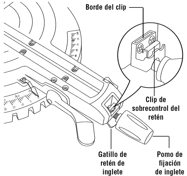
Figura 24. Sobrecontrol del retén
