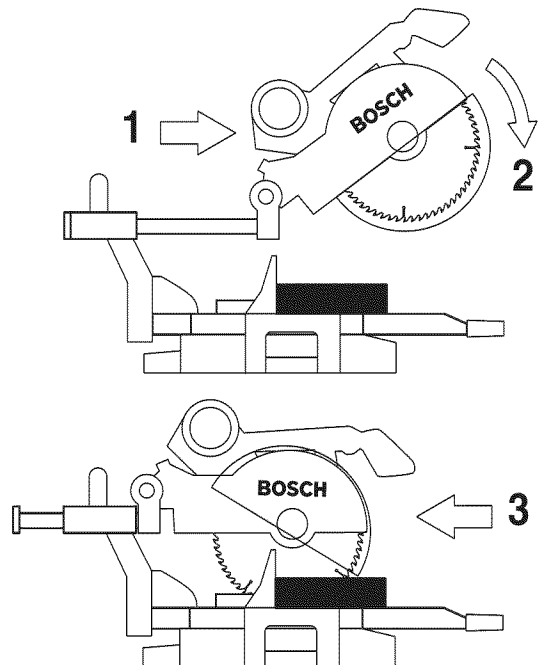
Figura 27. Corte deslizante
