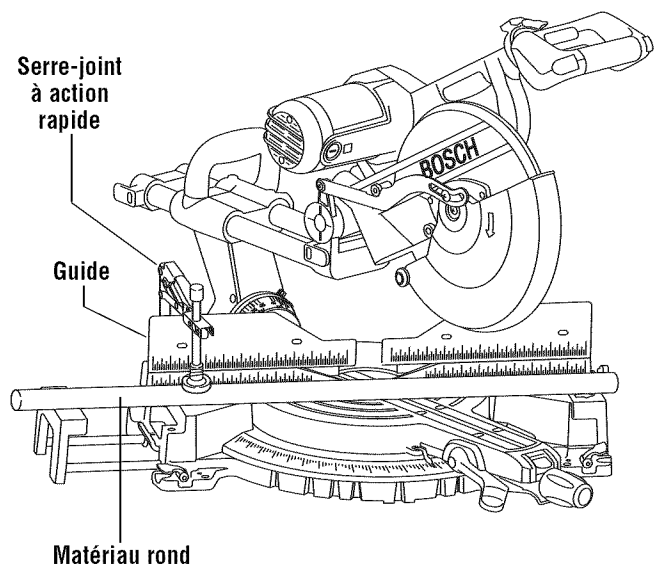
Figure 38. Matériau rond
