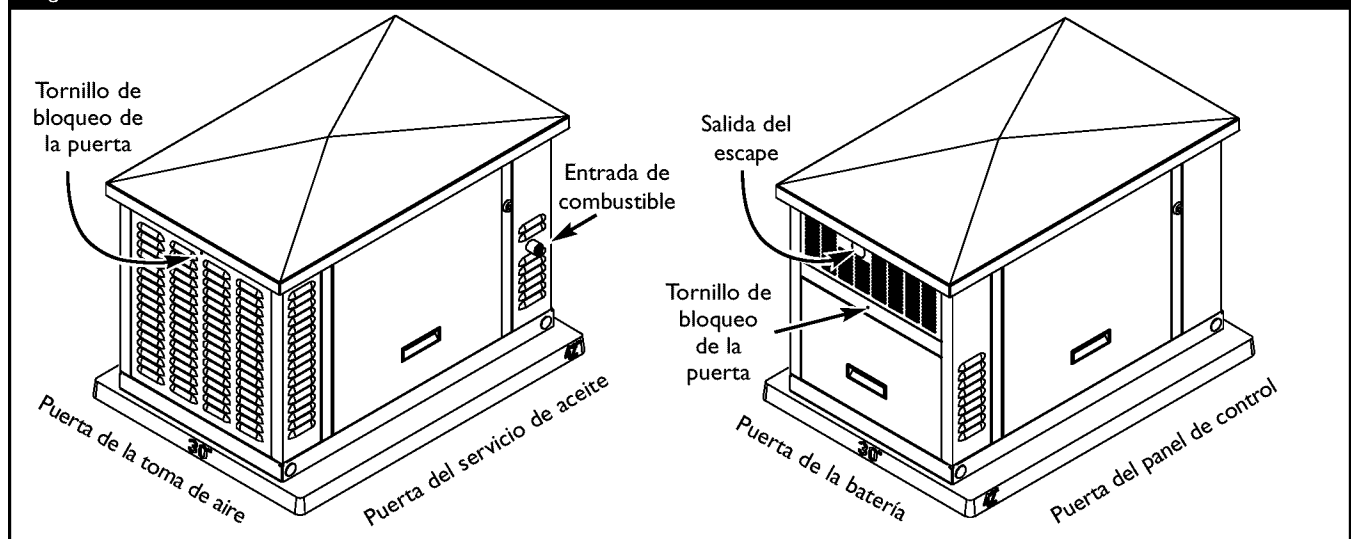
Figura 8 — Puertas de Acceso
