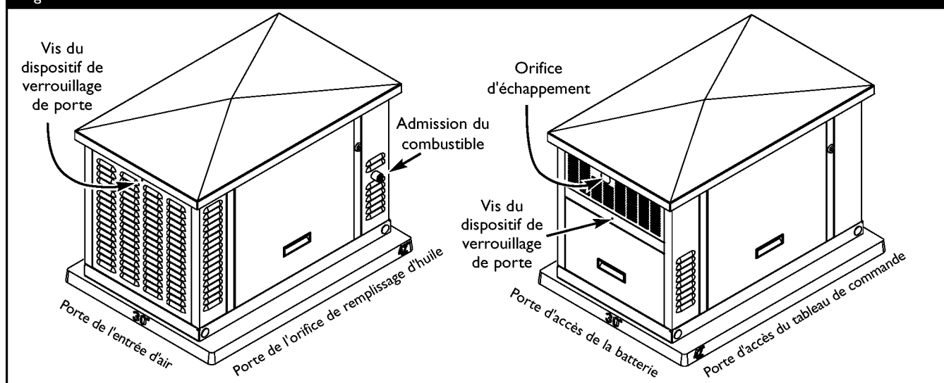
Figure 13 — Portes d'Accès de l'Enceinte
