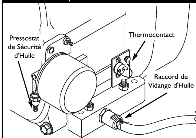
Figure 12 — Faible Pression d'Huile et Température Élevée Interrupteurs
