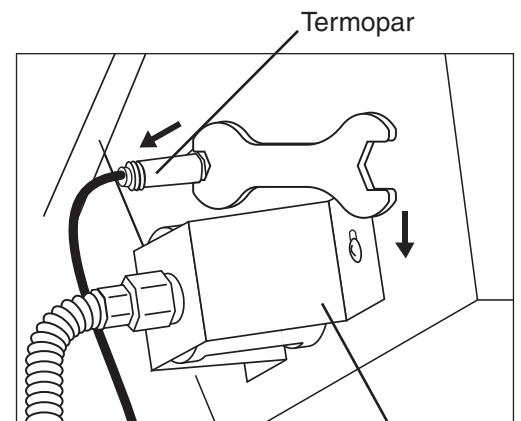
Válvula de la Hornilla para Dorar
