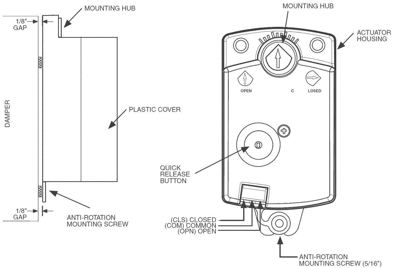
Fig. 4 – Actuator Detail
