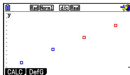
Color Link: OnlyX (gráfico de dispersión)
