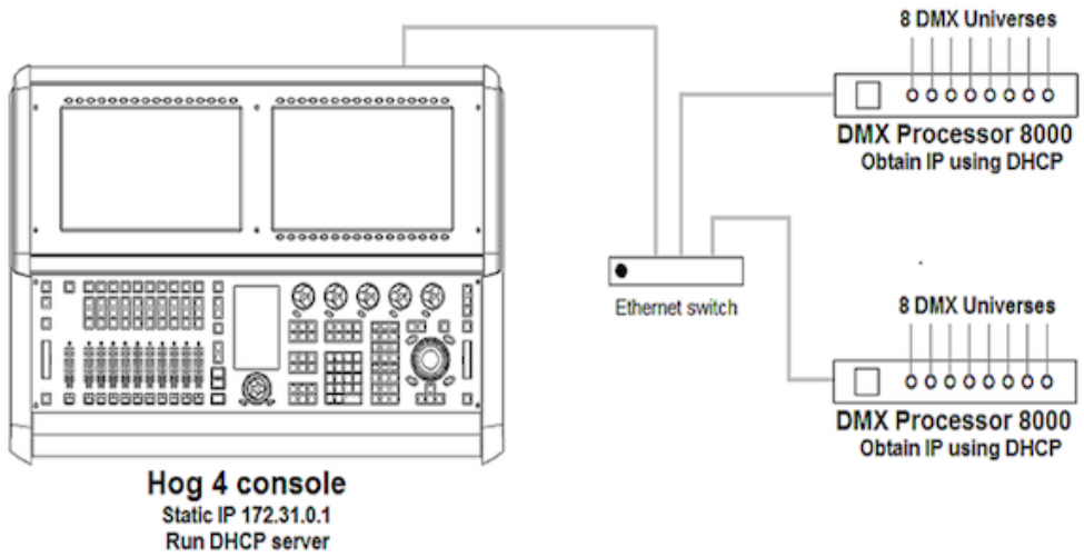
Exemple C: Un routeur DHCP fournit les adresses à toutes les machines.
