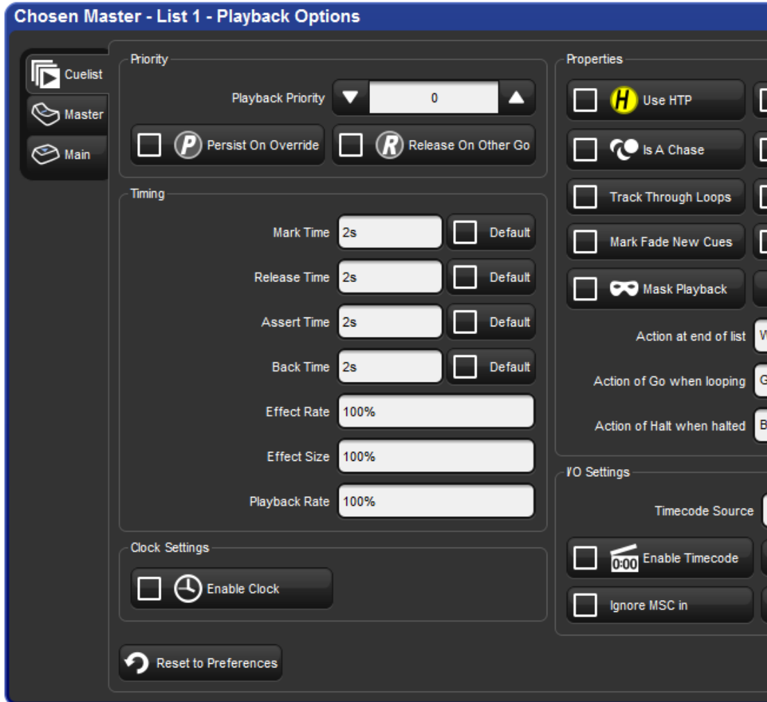
Figure 17.4. L'onglet Cuelist de la fenêtre Playback Options
