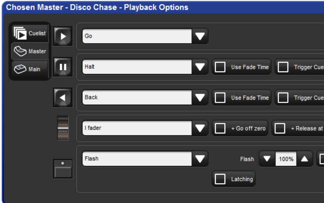
Figure 17.10. L'onglet Master de la fenêtre Cuelist Options
