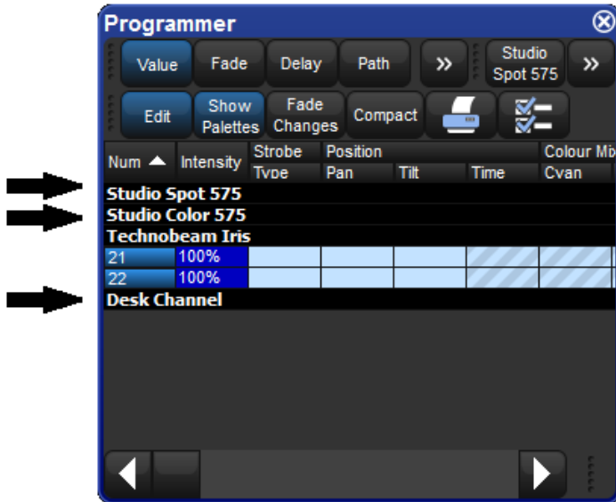
Figure 2.14. Un spreadsheet agrégé avec des lignes repliées
