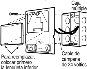
Figura 4 QUITAR LA TAPA
