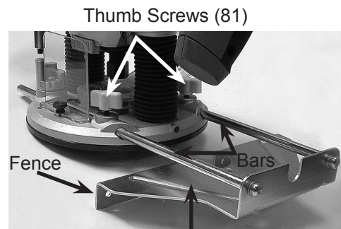
Figure 5 Edge Guide
