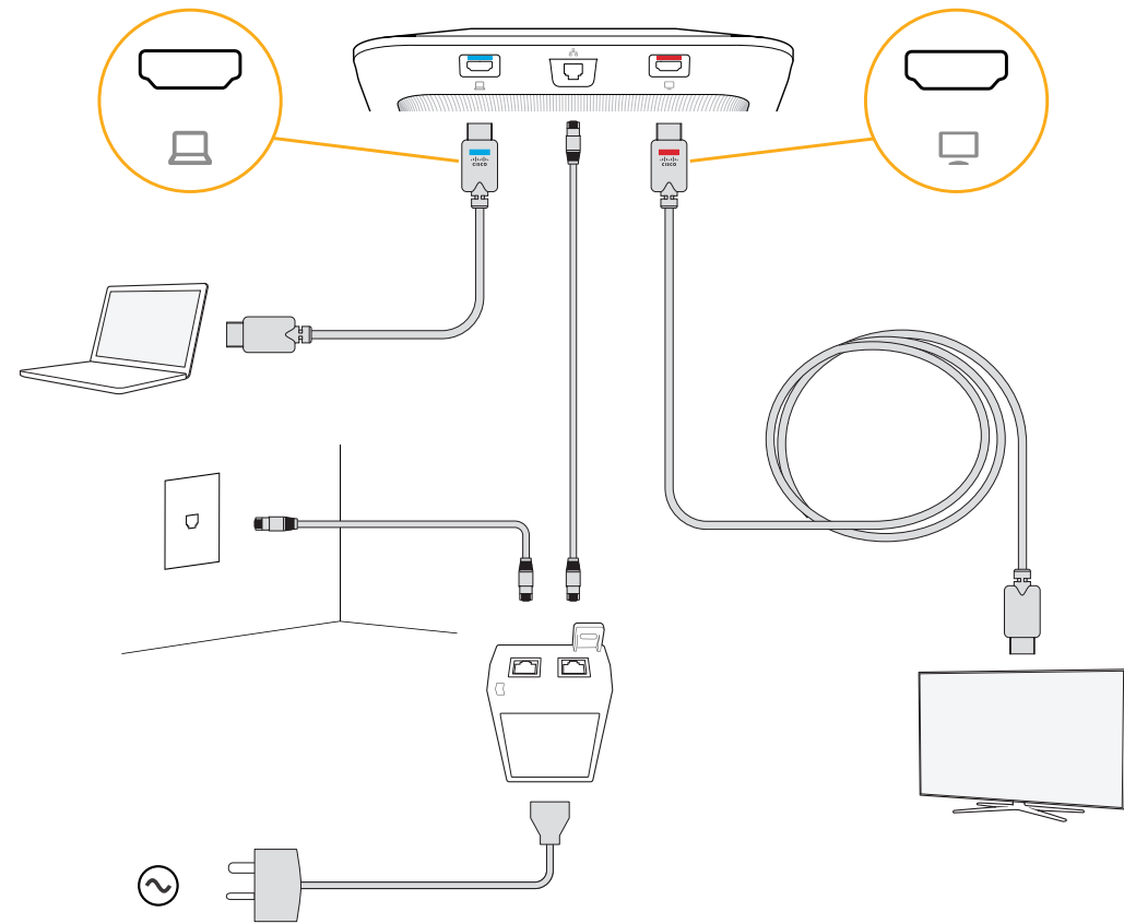
Ethernet with a power injector Ethernet avec injecteur de courant Ethernet mit einem Powerinjector Ethernet com um injetor de alimentação Ethernet con un inyector de alimentación Ethernet con iniettore di alimentazione
