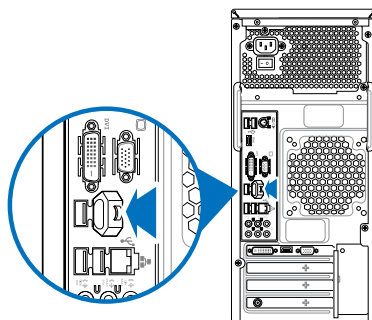
Pannello posteriore
