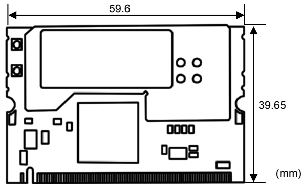
Figure1 : FX-DS540-MPCI4W
