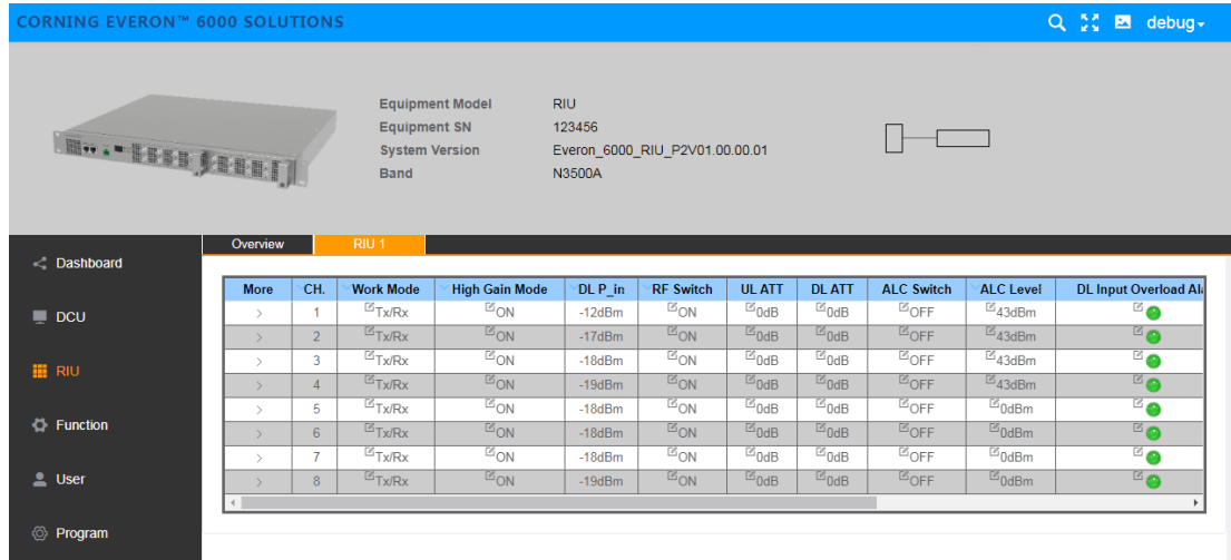
Figure 6.1-2 RIU WEB configuration page
