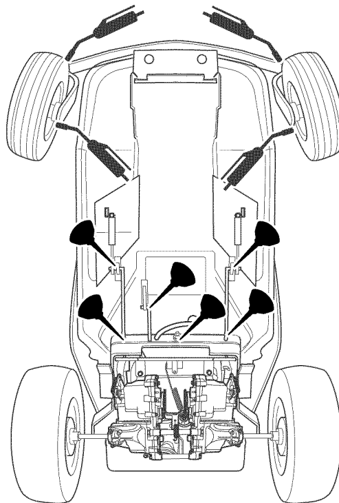
Figure 20. Lubricación del montable
