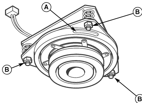
Figura 26. Ajuste del Embrague del PTO A. Ventana de Ajuste (Ctd. 3, se muestra una) B. Tuerca de Ajuste (3)
