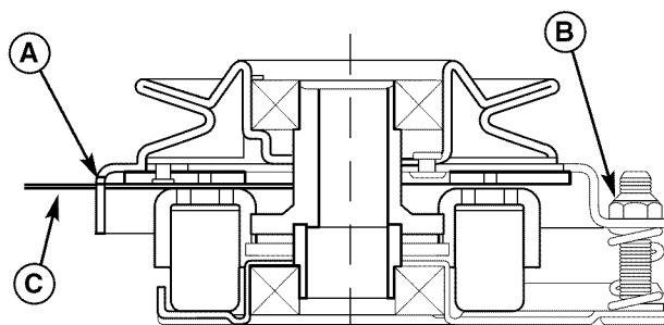
Figura 27. Ajustar Embrague del PTO A. Ventana B. Tuerca de Ajuste C. Lámina Calibradora
