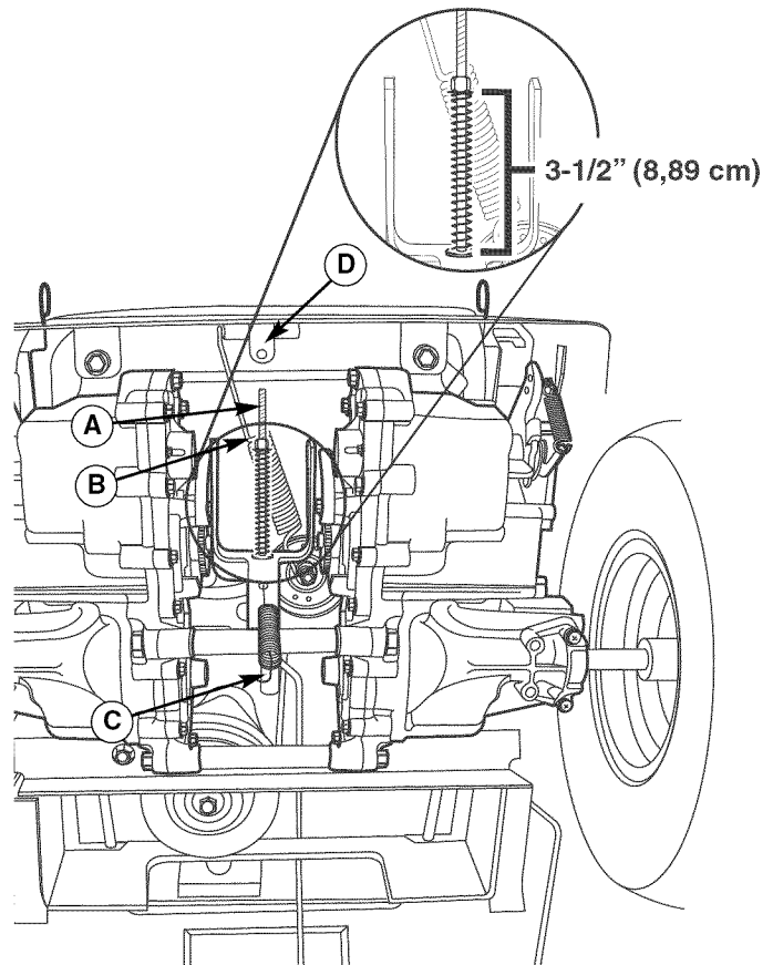
Figura 34. Ajuste del freno
