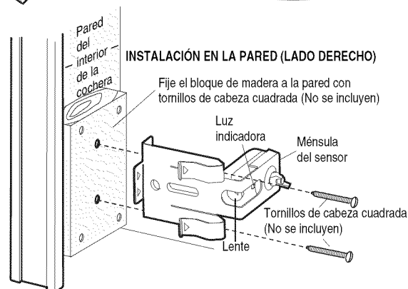
Figura 3 INSTALACIÓN EN LA PARED (LADO DERECHO)
