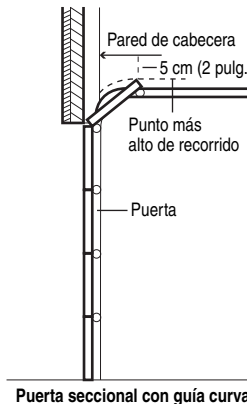
Puerta seccional con guía curva
