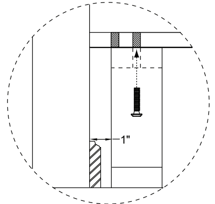
SIDE VIEW DETAIL VUE LATÉRALE – DÉTAILS DETALLE DE VISTA LATERAL
