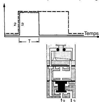
Générateur d'impulsion unique réglable
