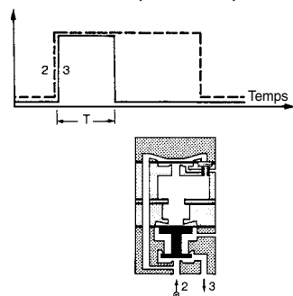
Générateur d'impulsion unique
