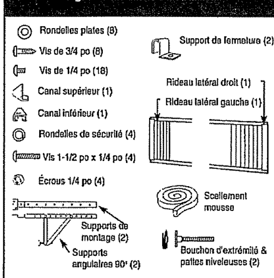
Fig. 1 Quincaillerie d'installation:
