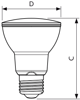
PAR20 120V 6W-50W 500lm 25D 2700K E26 D
