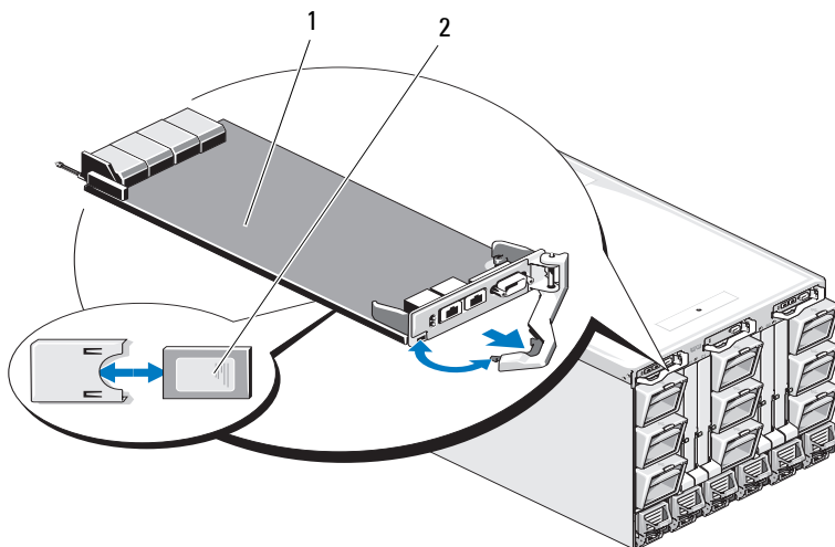
Ilustración 1-1. Cómo retirar e instalar una tarjeta SD del módulo CMC
