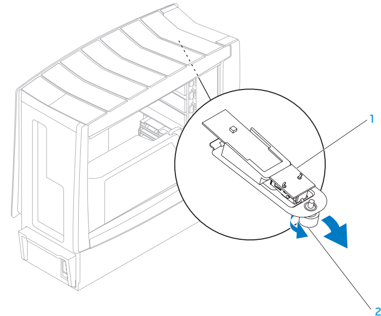
1 Bluetooth module
