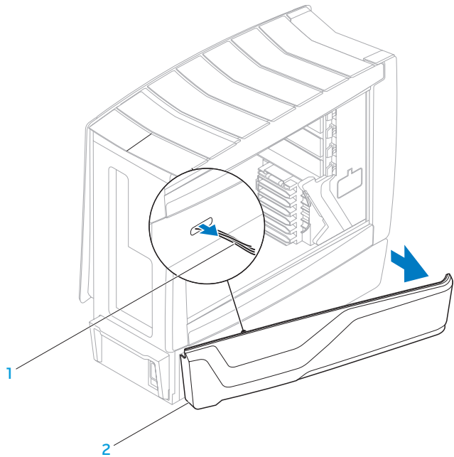
1 left bottom-panel cable
