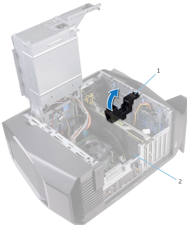
Рисунок 27. Извлечение видеокарты
