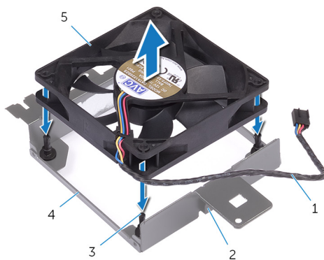
Рисунок 40. Снятие верхнего вентилятора корпуса
