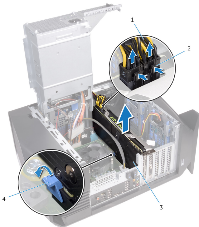
Рисунок 28. Извлечение видеокарты
