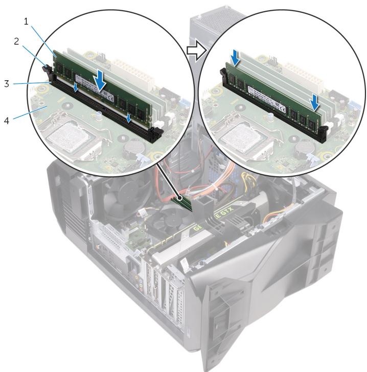
Рисунок 26. Установка модуля памяти
