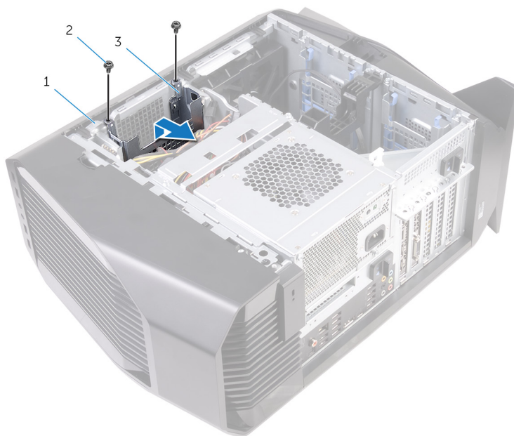
Figura 17. Rimuovere la gabbia del disco rigido
