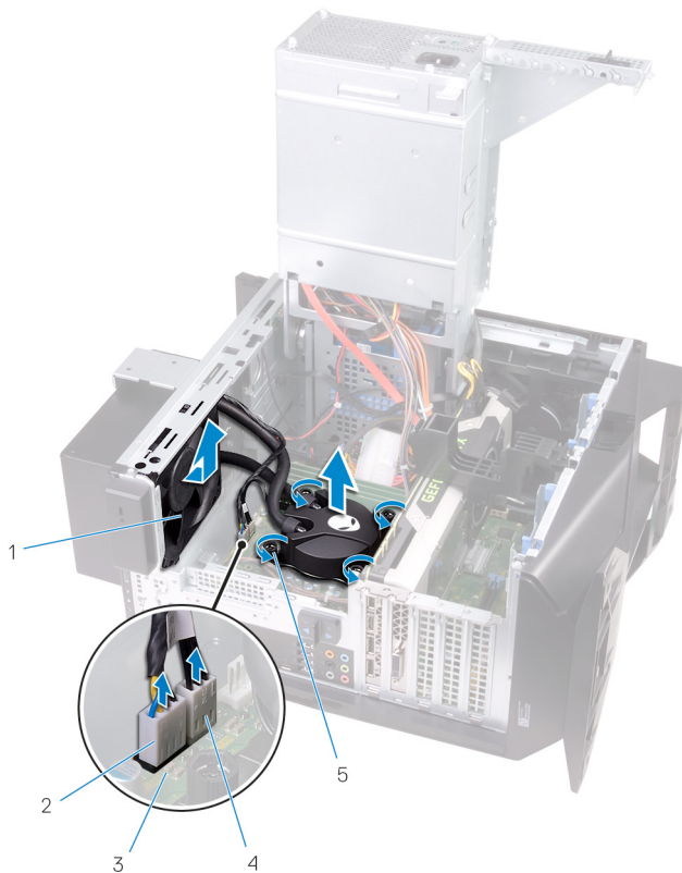
Figura 21. Rimozione del gruppo di raffreddamento del processore
