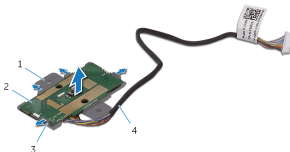
Figura 48. Rimozione del modulo di Accensione
