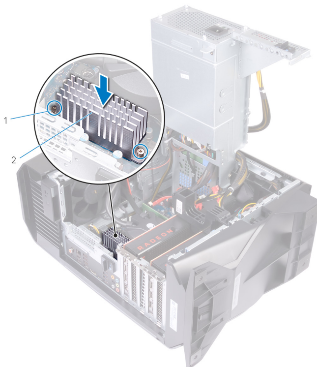
Figura 23. Ricollocamento del dissipatore di calore VR
