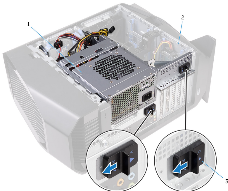
Figura 18. Far scorrere le chiusure a scatto della gabbia dell'unità di alimentazione
