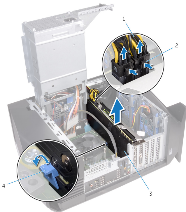
Figura 28. Rimozione della scheda grafica
