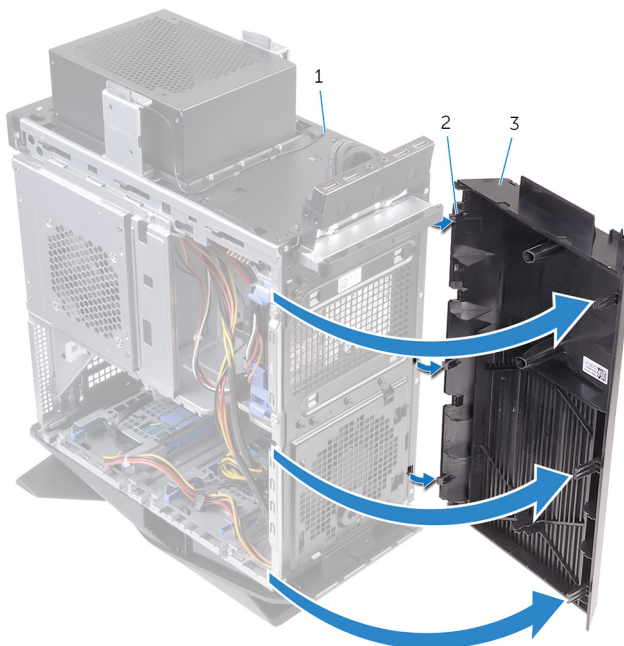
Figura 46. Rimozione del frontalino anteriore
