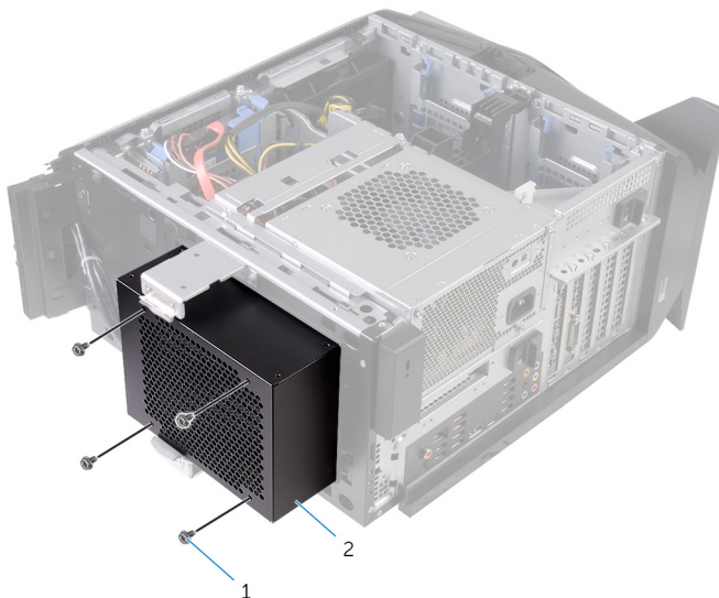
Figura 19. Rimozione del gruppo di raffreddamento del processore
