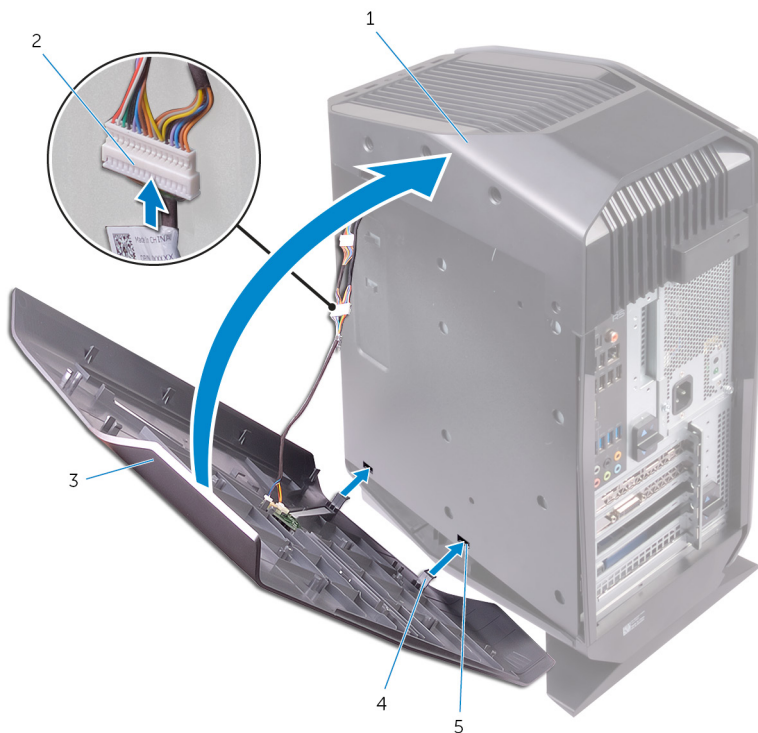
Figura 6. Collegare il cavo di illuminazione
