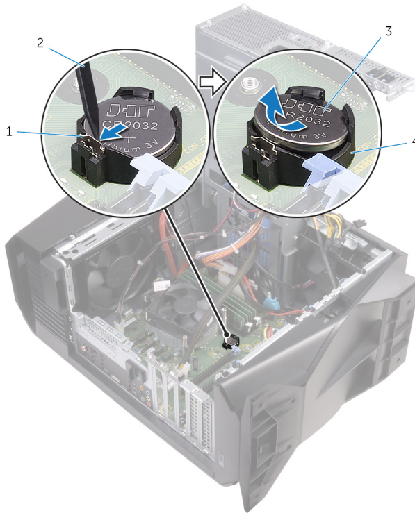
Figura 24. Rimozione della batteria pulsante
