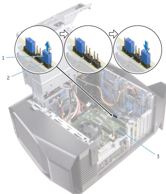
Figura 52. Cancellazione delle password dimenticate
