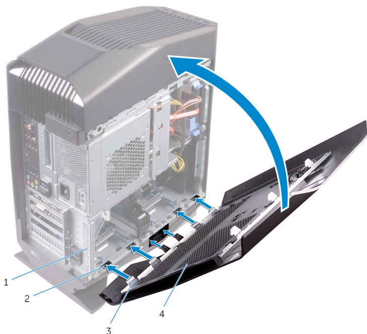
Figura 3. Ricollocamento del pannello laterale sinistro
