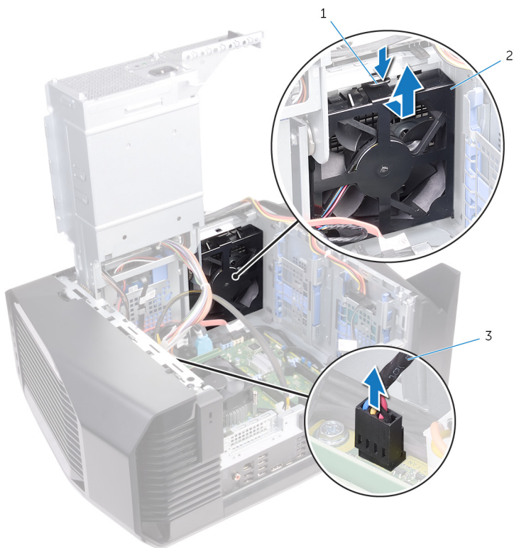
Figura 37. Rimozione della ventola del telaio
