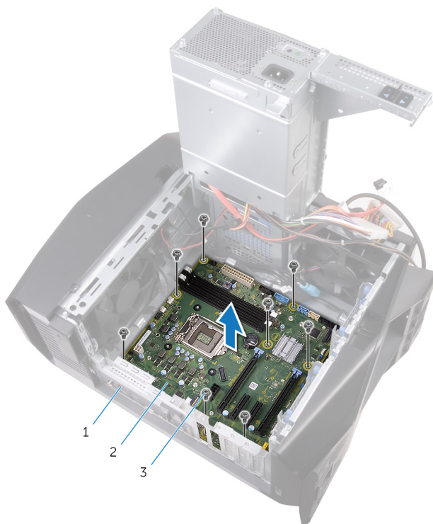
Figura 51. Rimozione della scheda di sistema
