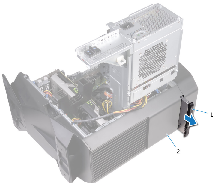
Figura 42. Rimozione dell'unità ottica
