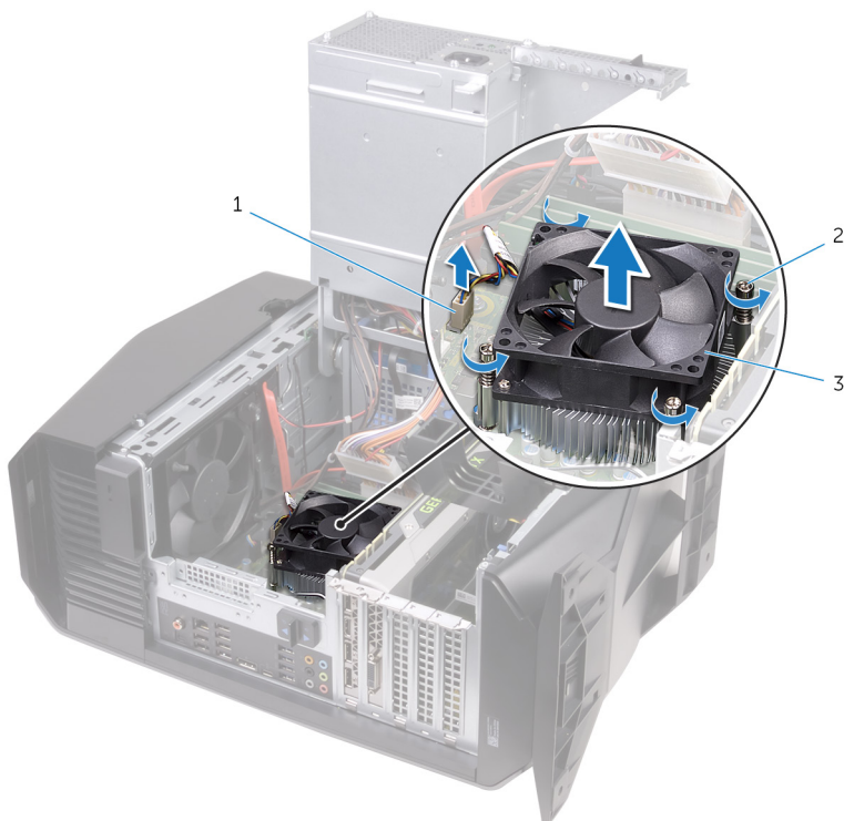
Figura 30. Rimuovere il gruppo ventola del processore e dissipatore di calore
