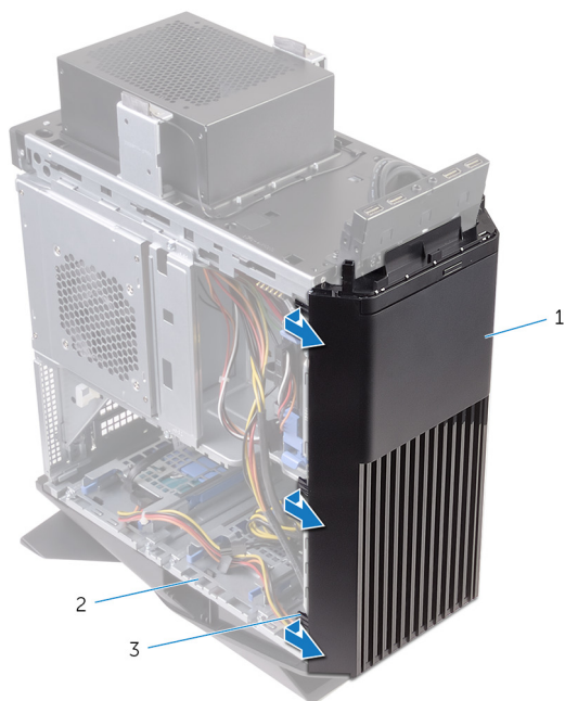
Figura 45. Rimozione del frontalino anteriore
