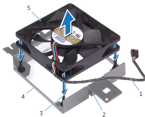
Figura 40. Rimozione della ventola superiore dallo chassis
