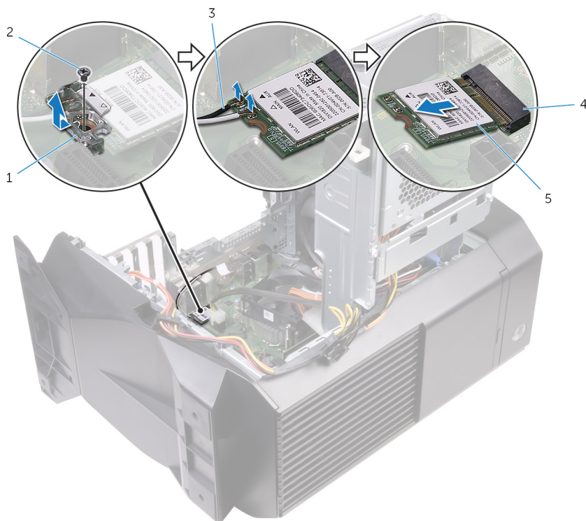
Figura 33. Rimozione della scheda per reti senza fili
