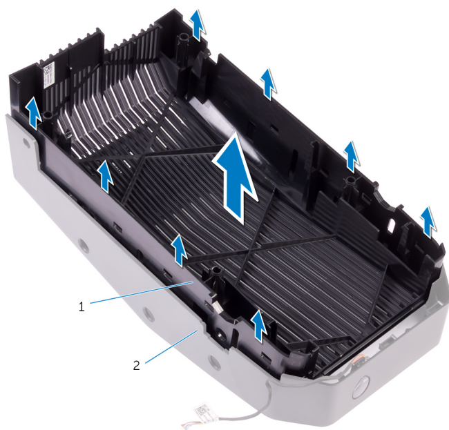
Figura 11. Sollevare il coperchio superiore dalla cornice superiore.
