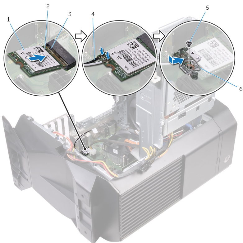
Figura 34. Ricollocamento della scheda per reti senza fili.
