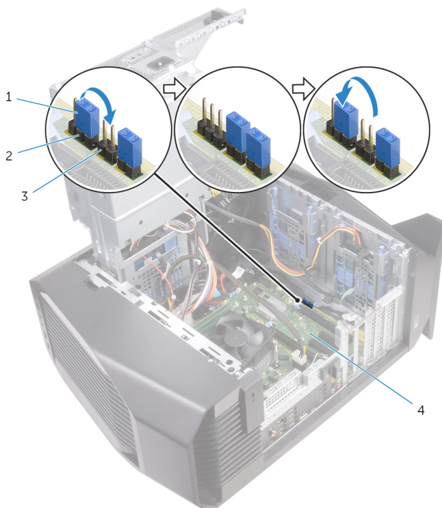
Figura 53. Cancellazione delle impostazioni CMOS
