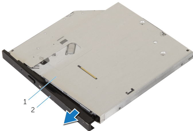
Figura 44. Rimozione dell'unità ottica
