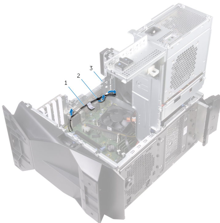
Figura 35. Rimuovere i cavi dell'antenna
