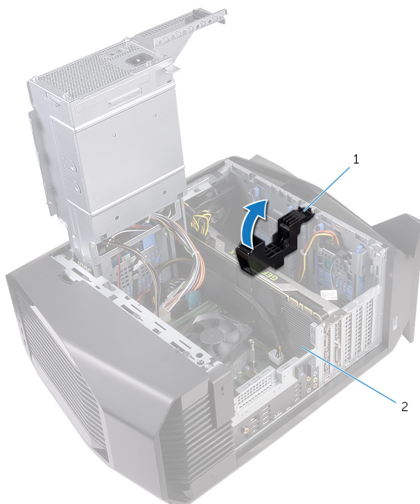
Abbildung 27. Entfernen der Grafikkarte
