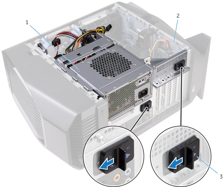
Abbildung 18. Schieben der Freigaberiegel des Netzteilgehäuses
