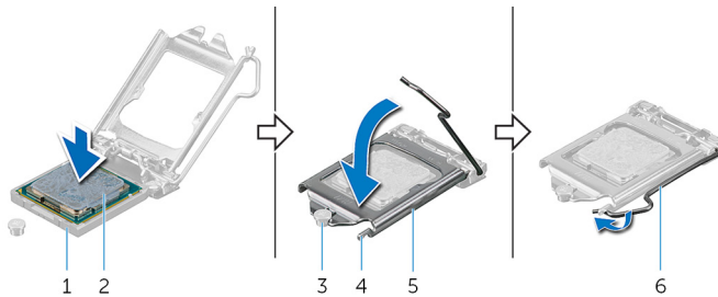
Abbildung 32. Einsetzen des Prozessors
