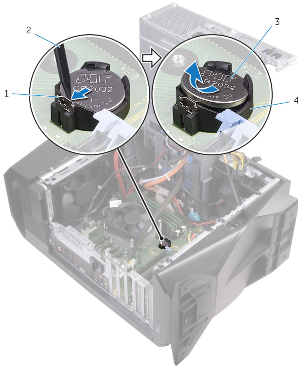
Abbildung 24. Entfernen der Knopfzellenbatterie
