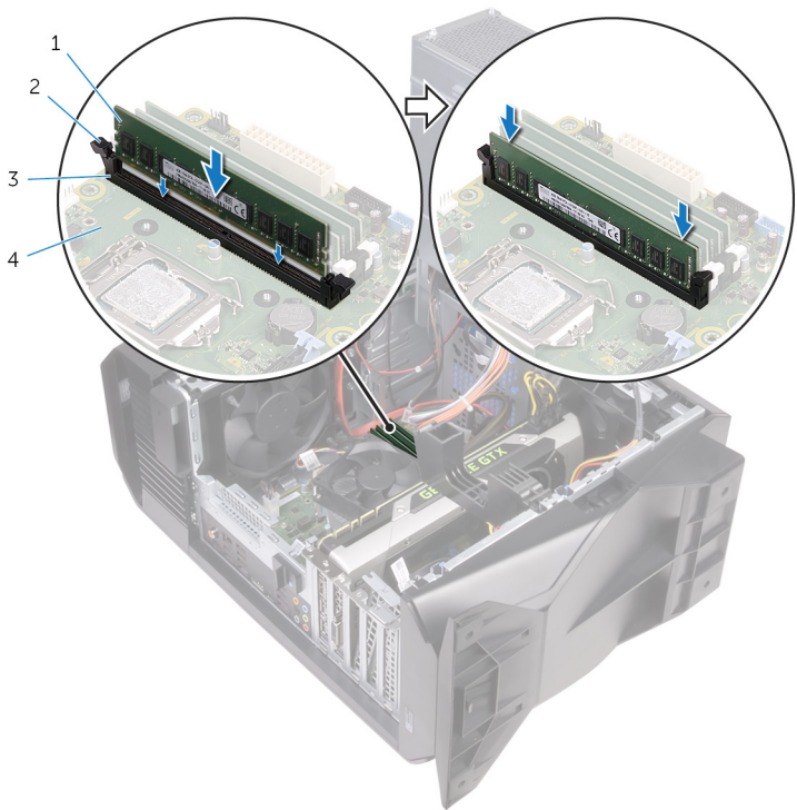
Abbildung 26. Austauschen des Speichermoduls
