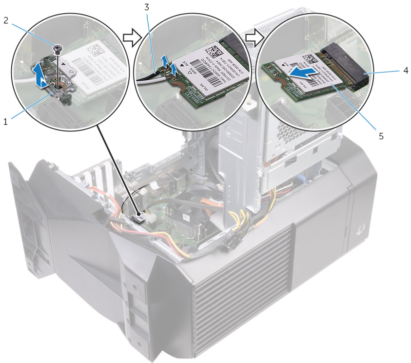
Abbildung 33. Entfernen der Wireless-Karte
