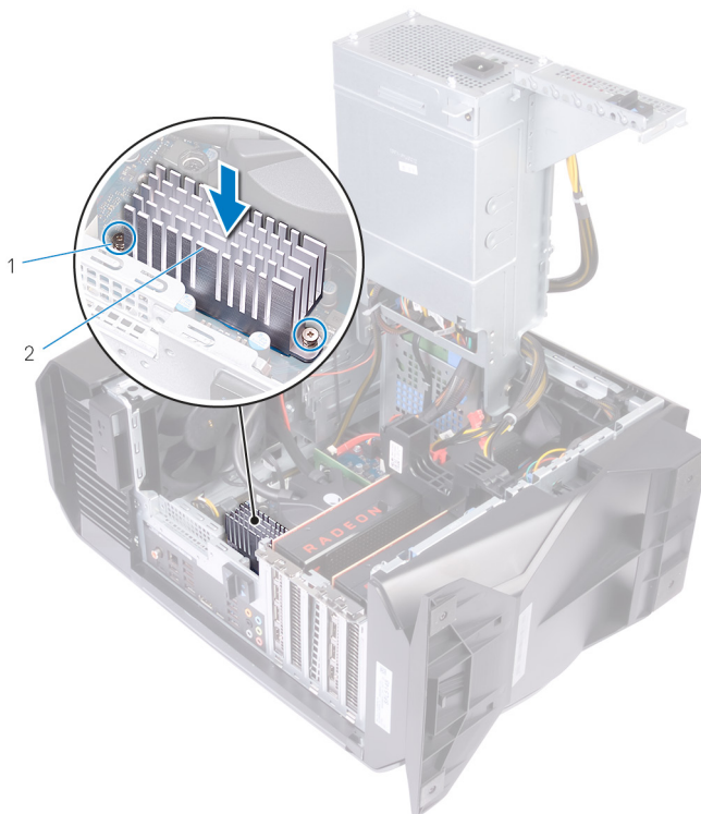
Abbildung 23. Wiedereinbauen des VR-Kühlkörpers
