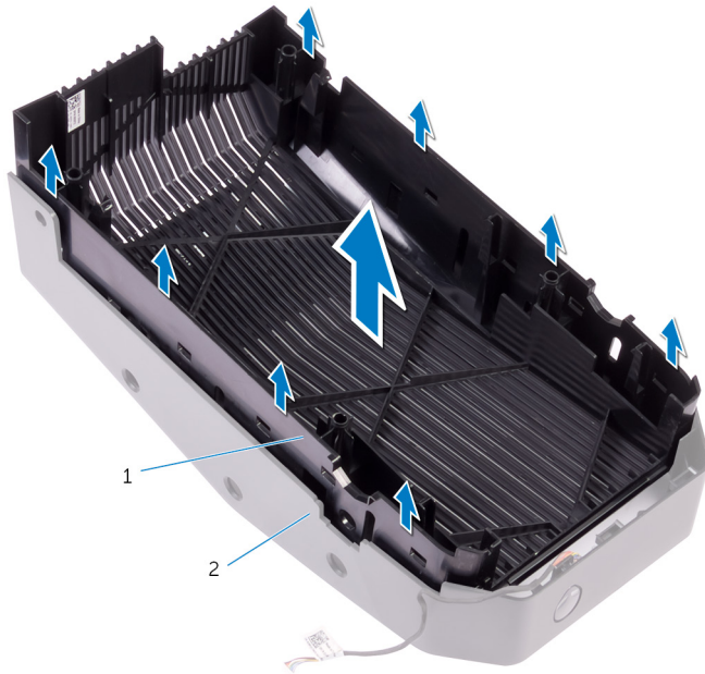
Abbildung 11. Abheben der oberen Abdeckung von der oberen Blende
