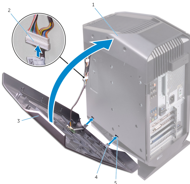
Abbildung 6. Anschließen des Beleuchtungskabels
