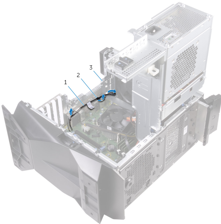
Abbildung 35. Entfernen der Antennenkabel
