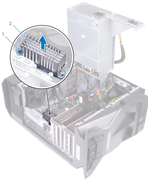
Abbildung 29. Entfernen des VR-Kühlkörpers
