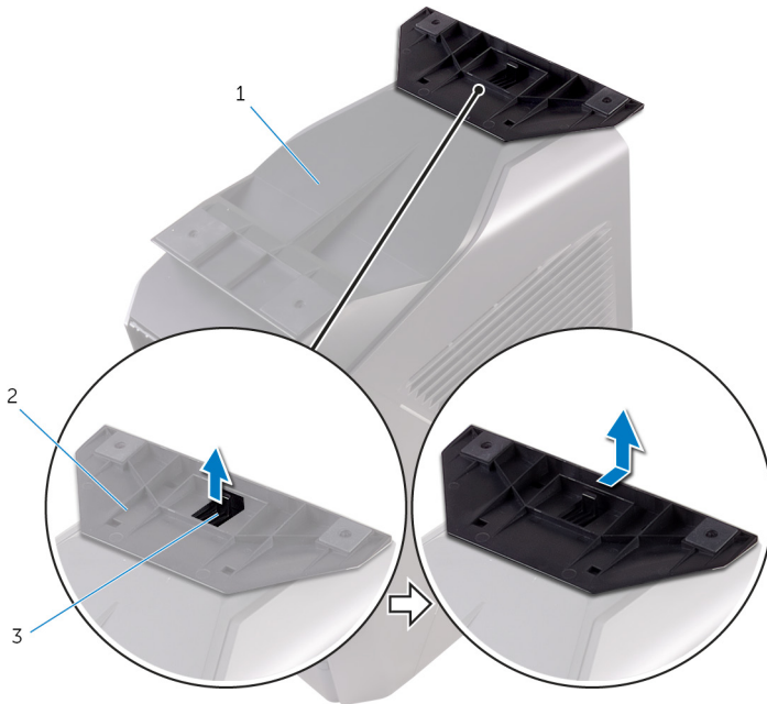
Abbildung 1. Entfernen des Standfußes
