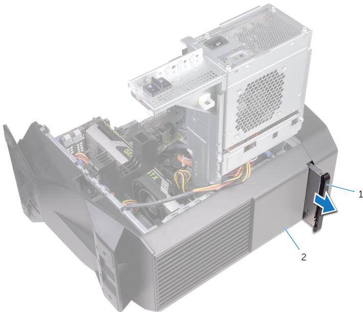
Abbildung 42. Entfernen des optischen Laufwerks
