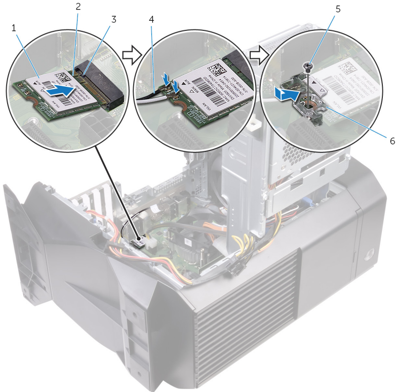
Abbildung 34. Wiedereinbauen der Wireless-Karte
