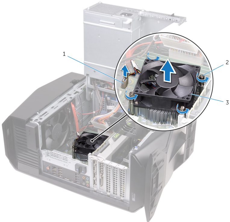
Abbildung 30. Entfernen der Prozessorlüfter- und Kühlkörperbaugruppe
