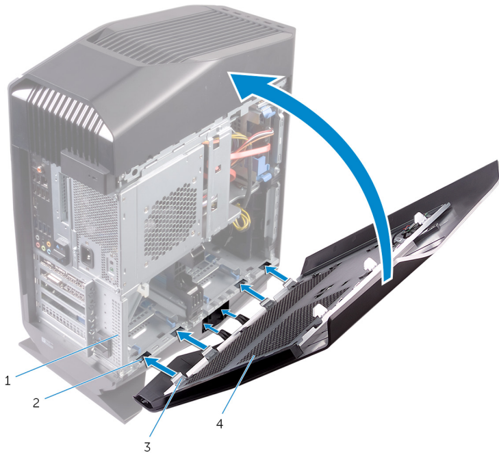
Abbildung 3. Ersetzen der linken Abdeckung
