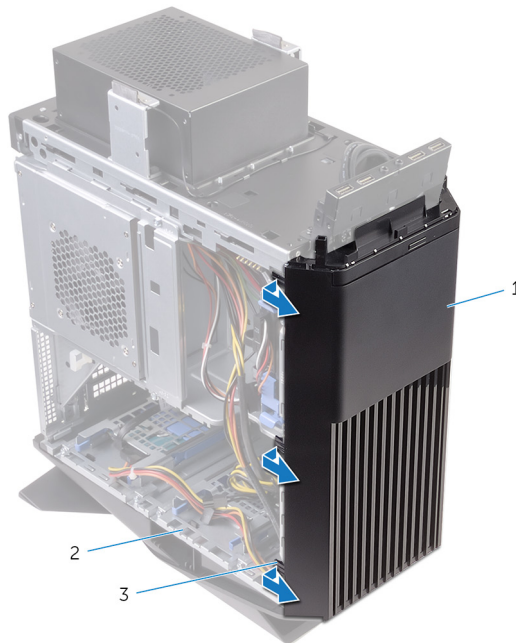
Abbildung 45. Entfernen der Frontverkleidung
