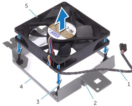
Abbildung 40. Entfernen des oberen Gehäuselüfters
