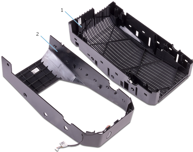
Abbildung 12. Obere Abdeckung und obere Blende
