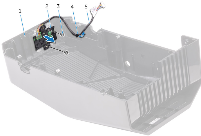
Abbildung 47. Entfernen des Betriebsschaltermoduls
