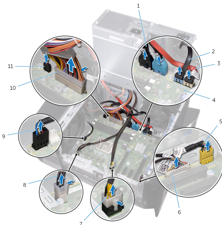
Abbildung 50. Entfernen der Systemplatine
