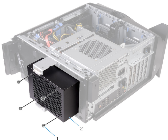
Abbildung 19. Entfernen der Prozessorkühlung-Baugruppe
