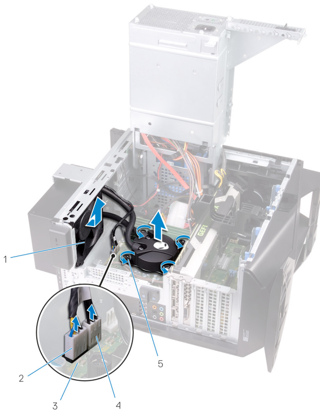
Abbildung 21. Entfernen der Prozessorkühlung-Baugruppe
