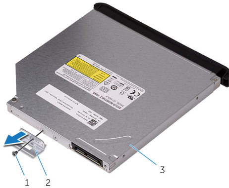
Abbildung 43. Entfernen des optischen Laufwerks
