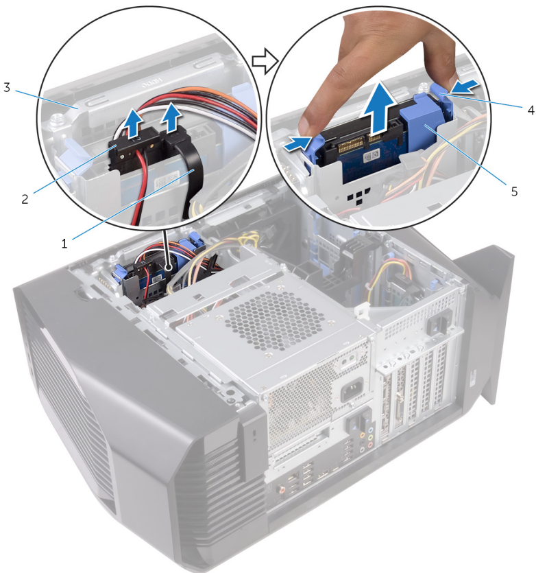
Abbildung 13. Entfernen des Festplattenlaufwerks
