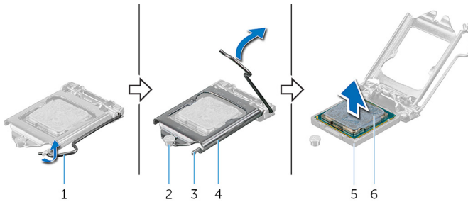
Abbildung 31. Entfernen des Prozessors
