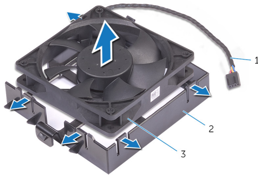
Abbildung 38. Entfernen des Gehäuselüfters
