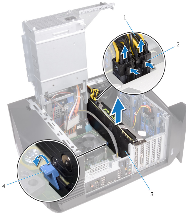
Abbildung 28. Entfernen der Grafikkarte
