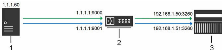
Ilustración 6. Diagrama de reenvío de puerto NAT iSCSI
