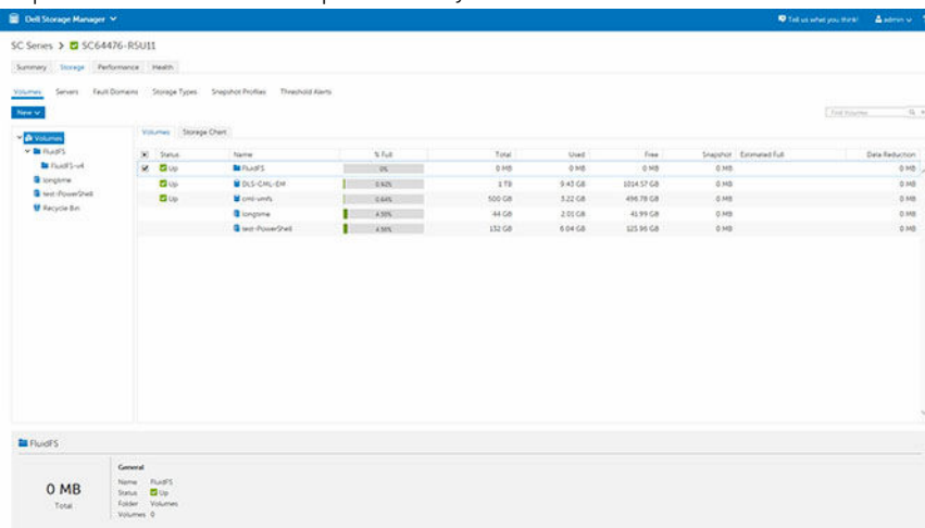
Ilustración 2. Pestaña Almacenamiento
