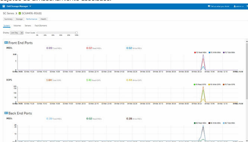
Ilustración 3. Pestaña Rendimiento
