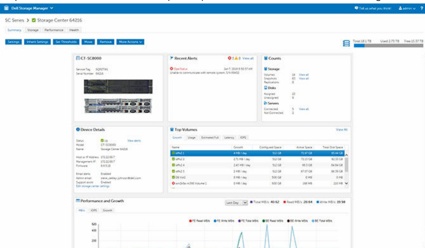
Ilustración 1. Pestaña Resumen
