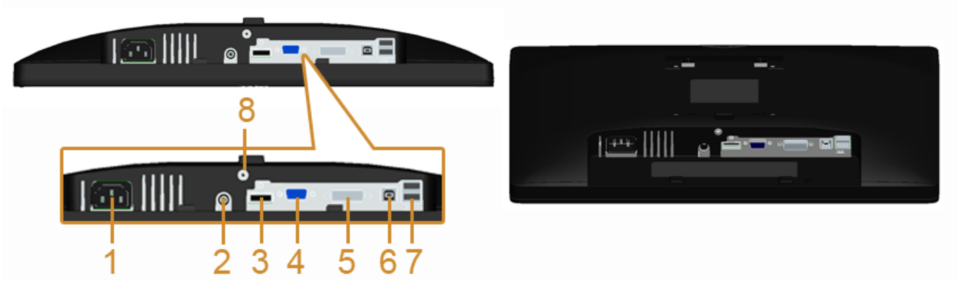
Tampilan bawah tanpa penyangga monitor
