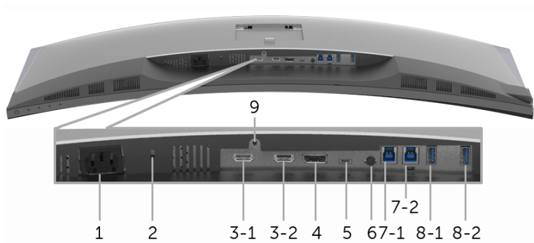
Ansicht von unten ohne Monitor-Standfuß
