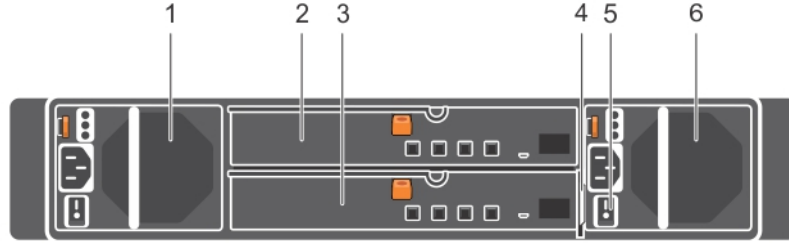
图 19: SCv300 和 SCv320 扩展柜背面板功能部件和指示灯
