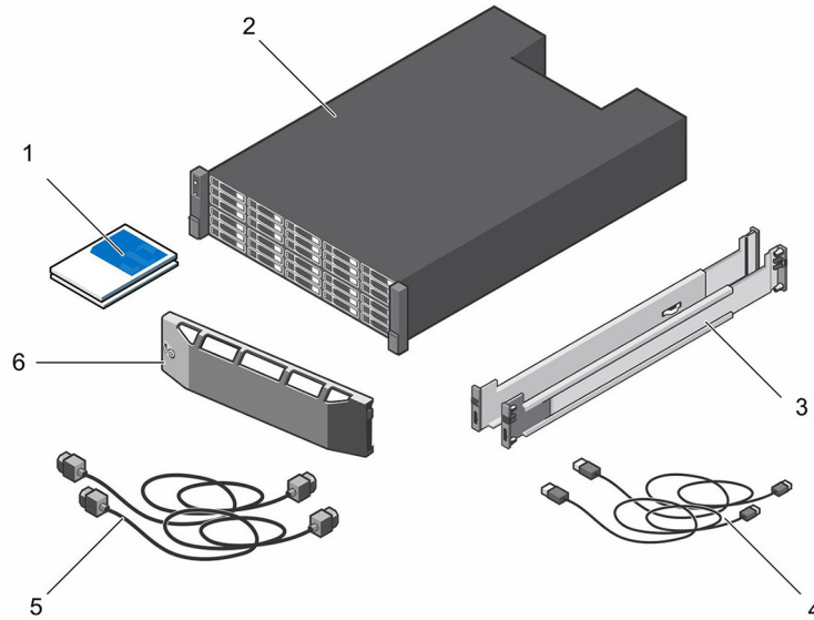
图 26: SCv3000 和 SCv3020 存储系统组件
