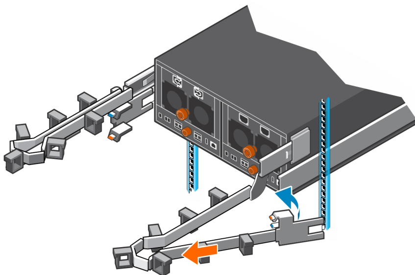
图 72: 将扩展臂与滑轨支架对齐
