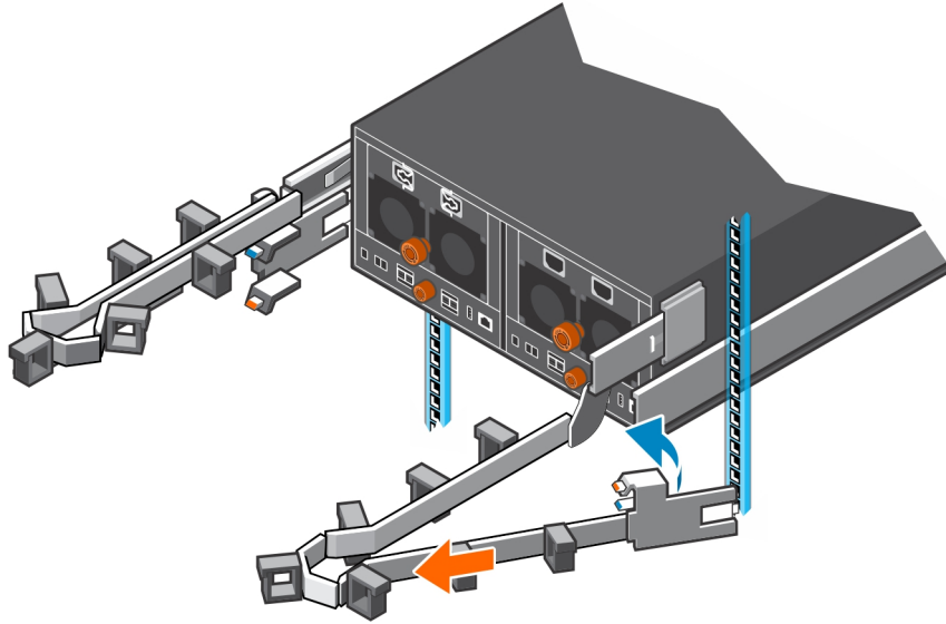
图 22: 将扩展臂与滑轨支架对齐
