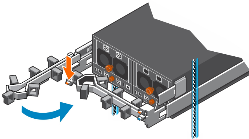
图 75: 向机箱右侧摆动上臂并固定下臂
