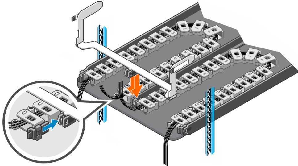
图 50: 从机箱支架断开电缆链
