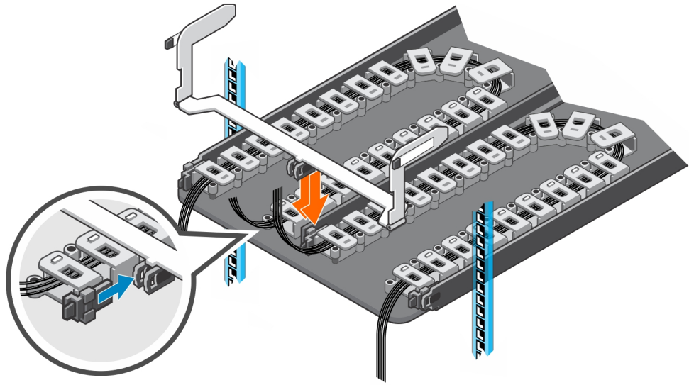
图 64: 将电缆链固定到机箱支架
