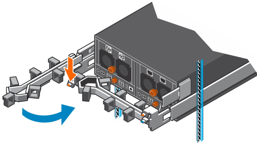
图 25: 向机箱右侧摆动上臂并固定下臂
