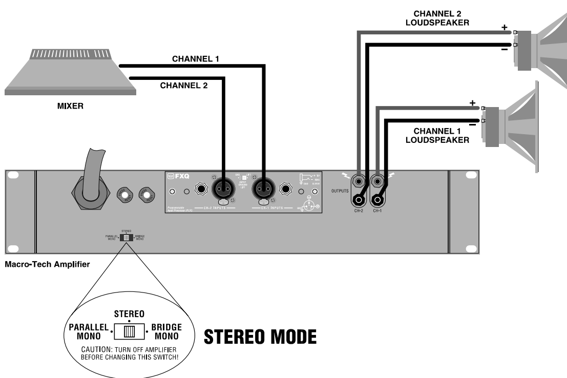
Fig. 3.4 Stereo Wiring
