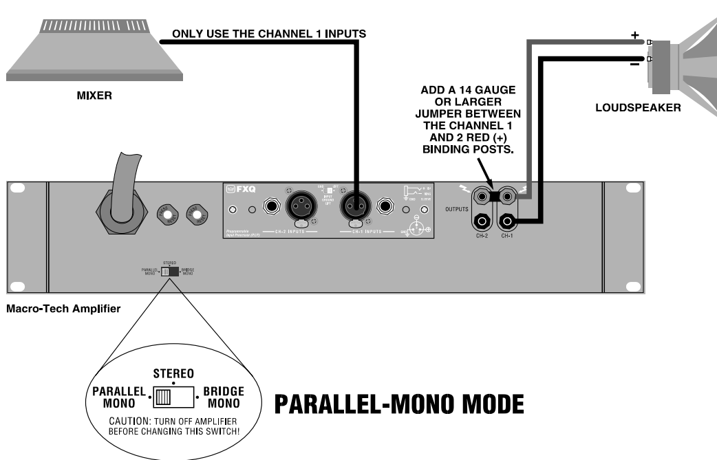
Fig. 3.6 Parallel-Mono Wiring
