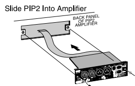
Fig. 8.3 Installing a PIP2 Module
