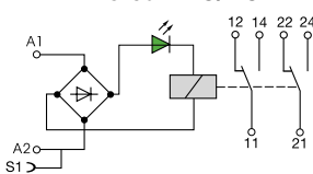
RB...122 A 115-230 V AC/DC
