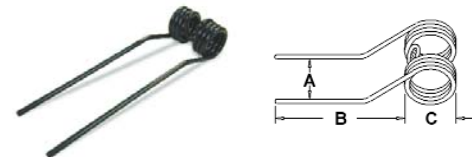
A-VLH7001 Rake & Tedder tooth
