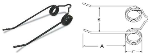
A-186SE Rake tooth
