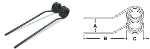
A-10370000 Rake & Tedder tooth
