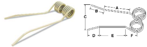
A-PZ225 Tedder tooth
