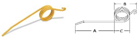
A-241380L LH Baler tooth
