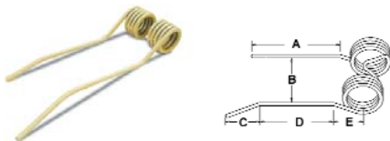
A-PZ224 Tedder Tooth
