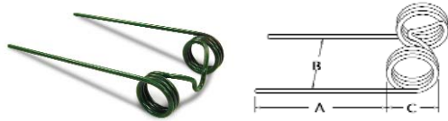
A-276SE Baler tooth
