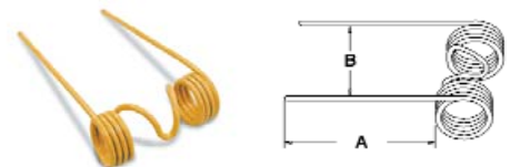
A-76517 Windrower teeth
