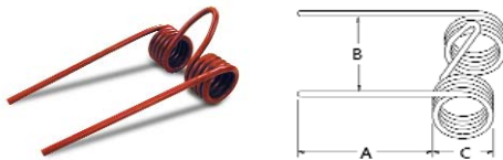
A-1711951 Baler tooth
