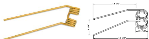
A-GS-3 LH Rake / Tedder tooth
