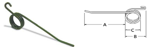
A-0782ME1 Rake teeth
