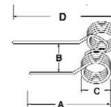
A-PZ339 Tedder Tooth (LH)
