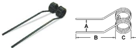
A-0946 TEDDER TOOTH
