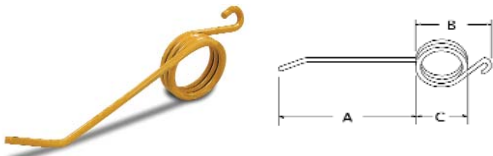
A-241379R RH Baler tooth
