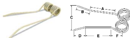
A-PZ225 Tedder Tooth
