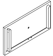
U. Top Drawer Front x2 Avant du Tiroir supérieur Parte frontal de la Gaveta superior #27458
