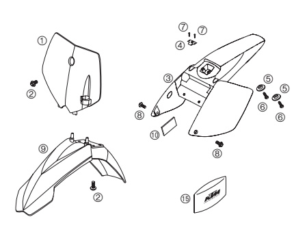
MASKE, KOTFLÜGEL MASK, FENDERS
