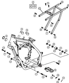
RAHMEN, AUSLEGER FRAME, SUB FRAME
