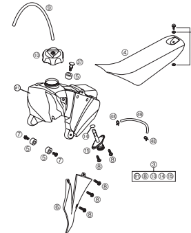
TANK, SITZBANK, VERKLEIDUNG TANK, SEAT, COVER
