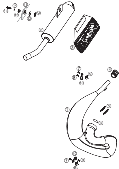
AUSPUFFANLAGE EXHAUST SYSTEM
