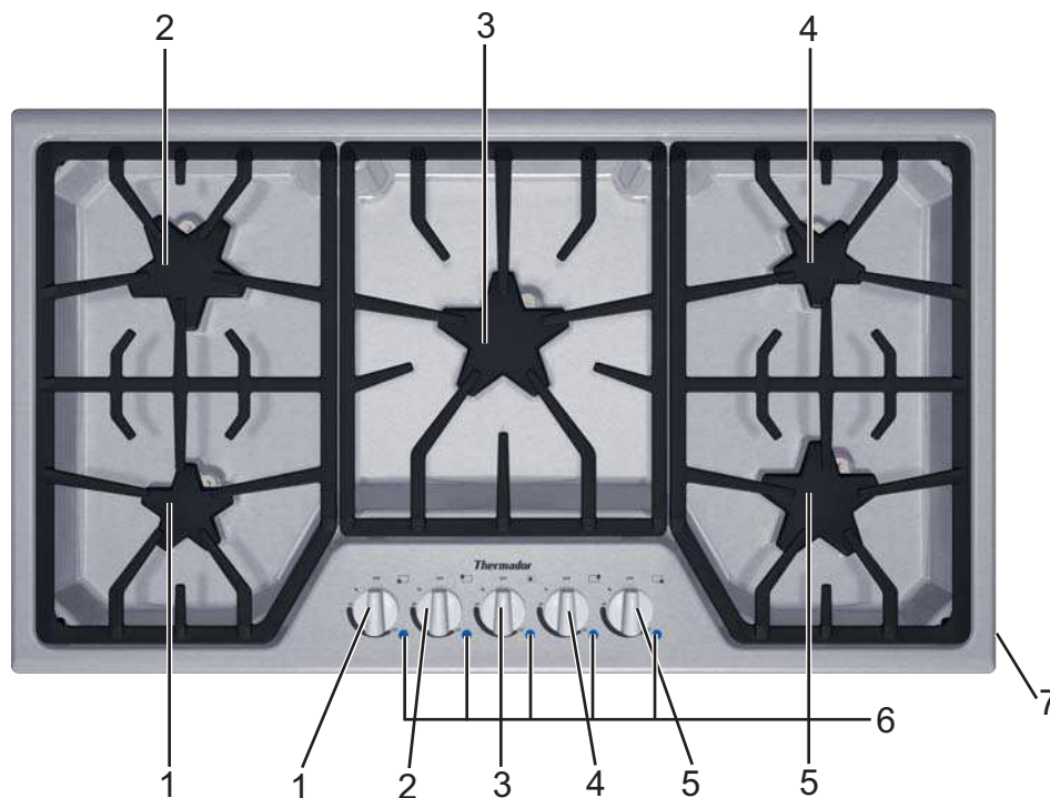
Figure 3: Modèle SGS365FS/SGSL365KS/SGSX365FS
