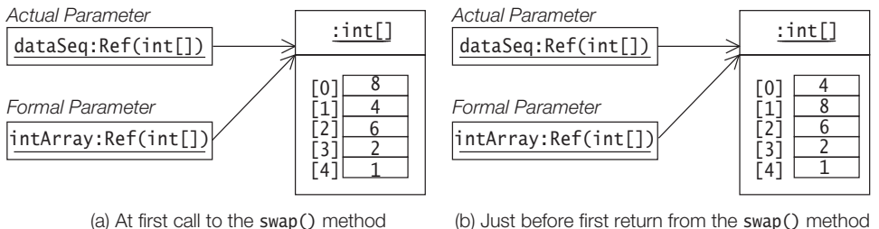
Figure 3.5 Parameter Passing: Arrays
