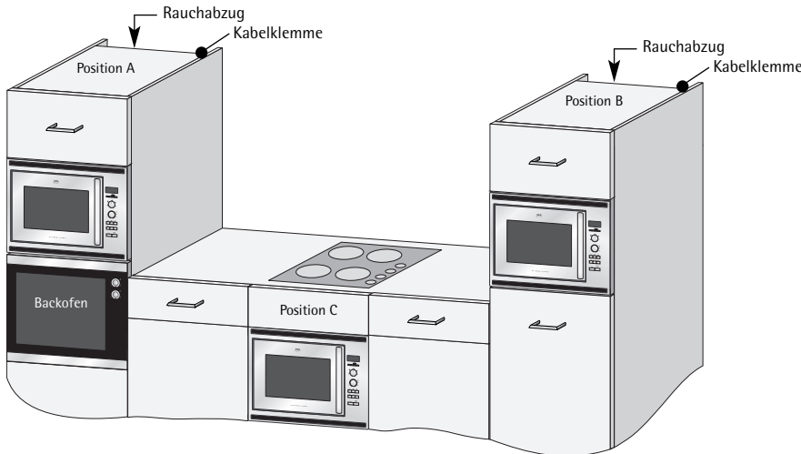
Die Mikrowelle kann in Position A, B oder C gepaßt werden:
