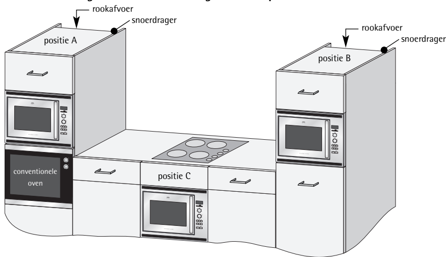
De magnetron kan worden ingebouwd in positie A ,B of C:
