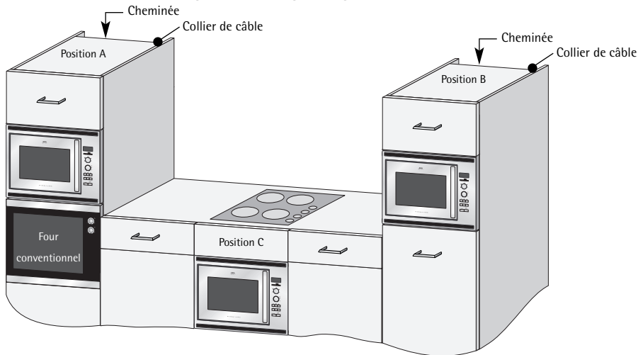
Le micro-onde peut être adapté en position A, B ou C :
