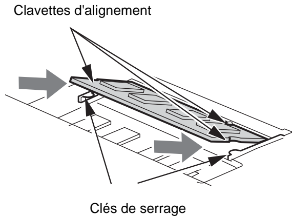
Figure 31. Installation du module de mémoire
