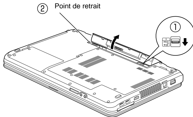
Figure 22. Retrait de la batterie
