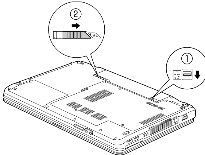
Figure 21. Verrou et loquet de la batterie
