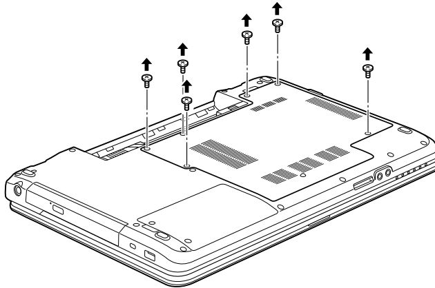
Figure 29. Retrait des vis du couvercle du module de mémoire
