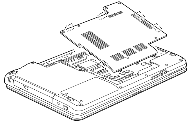
Figure 30. Retrait du couvercle du module de mémoire
