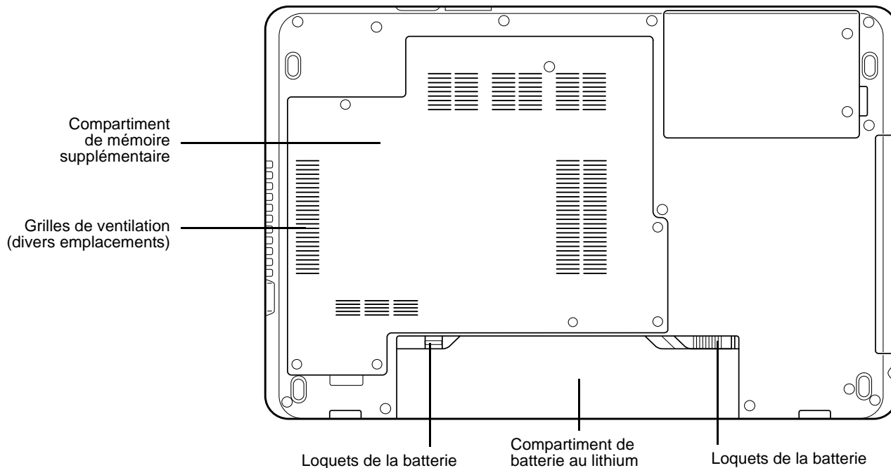
Figure 5. Dessous de l'ordinateur portable LIFEBOOK
