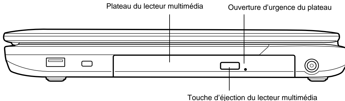
Figure 23. Lecteur optique
