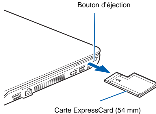
Figure 26. Installation/retrait d'une carte ExpressCard
