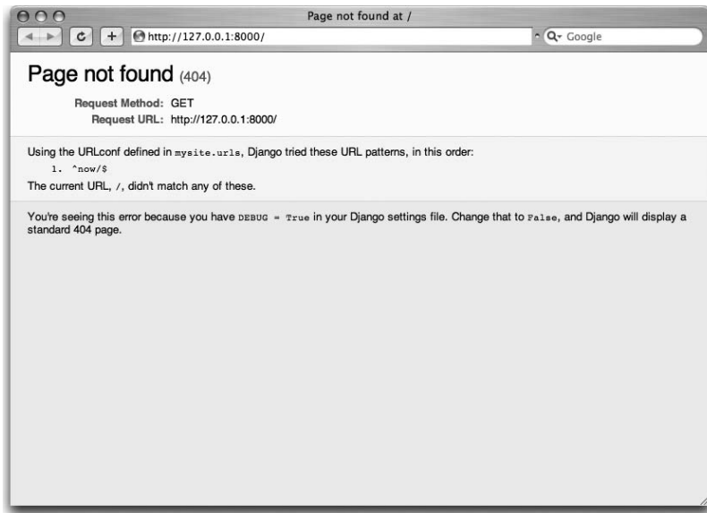
Figure 3-2. Django’s 404 page
