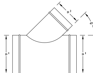
SP6276 45° LATERAL
