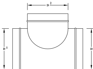
SP6271 90° TEE
