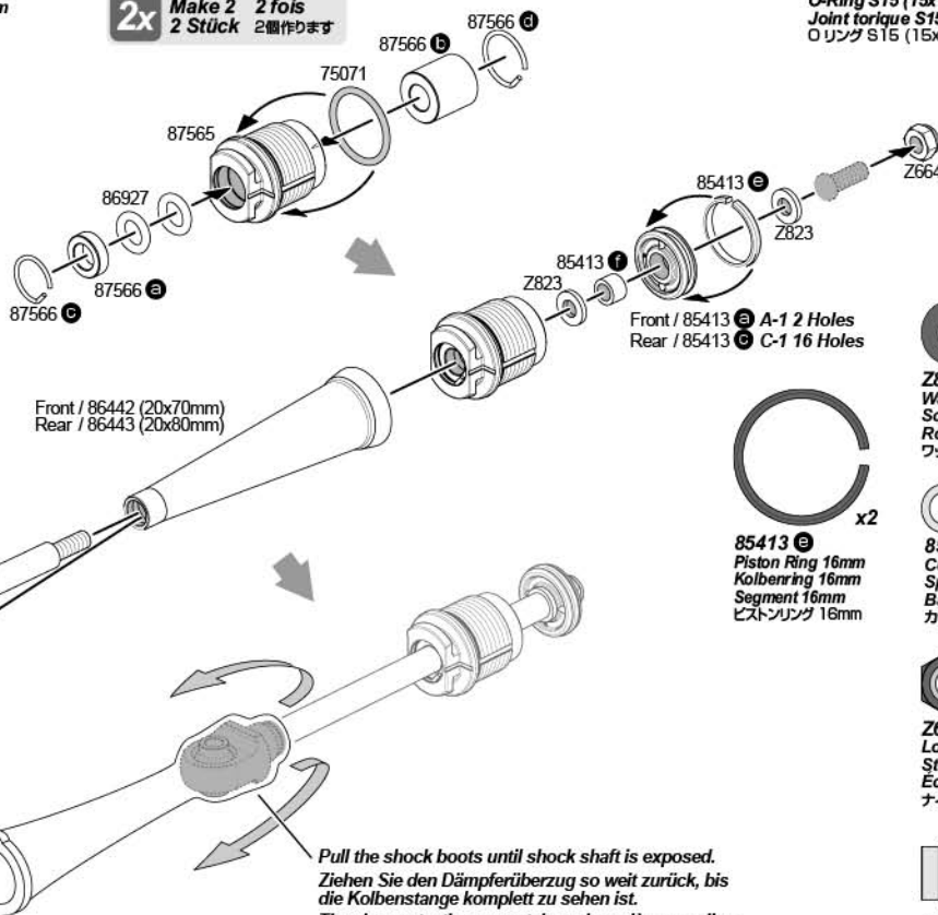
87566 b Metal Bushing 6x12x8mm Metall Lager 6x12x8mm Bague métal 6x12x8mm メタルブッシュ 6x12x8mm
