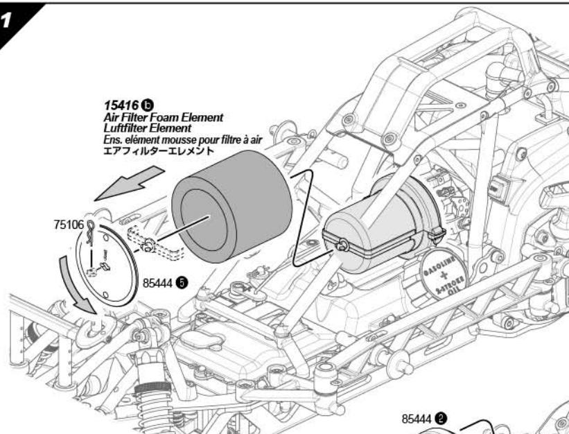
75106 Body Clip (6mm/Black) Karosserieklammer (6mm/Schwarz) Clip carr. (6mm/noir) ボディーピン (6mm/ブラック)
