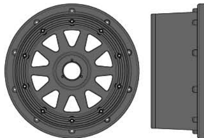
104975 TR-10 Wheel Black (120x60mm/-4mm Offset) TR-10 Felge Schwarz (120x60mm/vorne/-4mm Offset) Jante TR-10 Noire (120x60mm/deport -4mm) TR-10ホイールブラック (120x60mm/-4mmオフセット)
